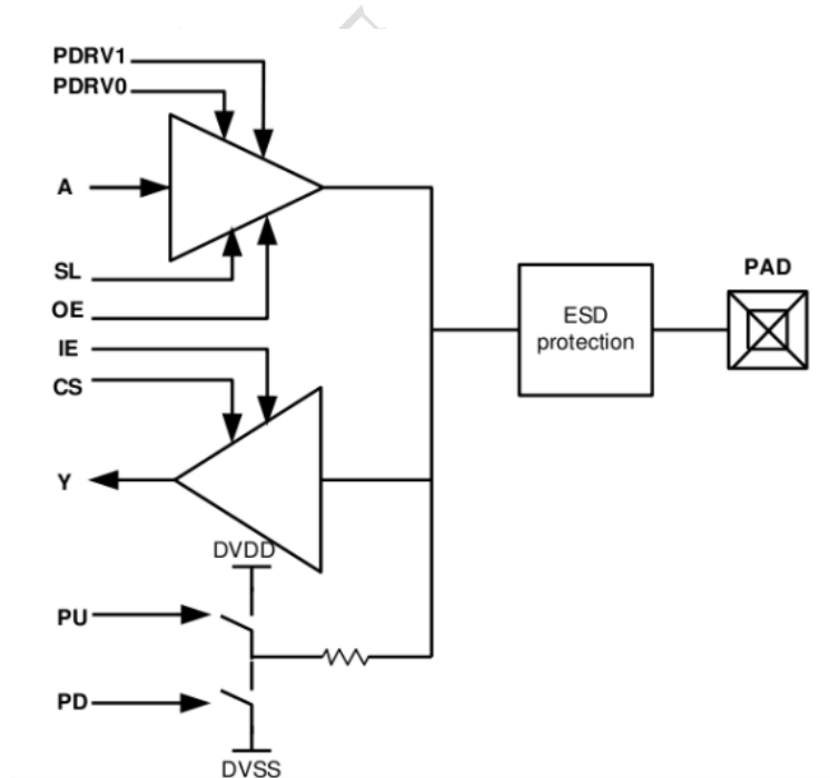
图 8 I/O 单元函数示意图
