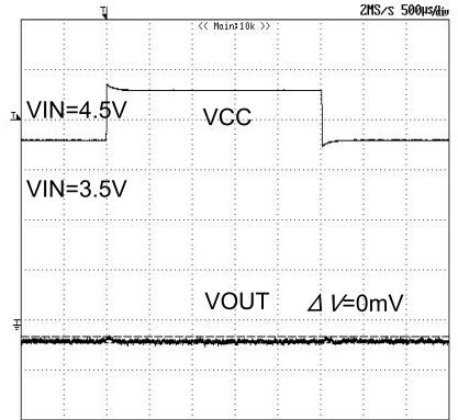
Fig.37 Transient_response (Ta=85°C)
