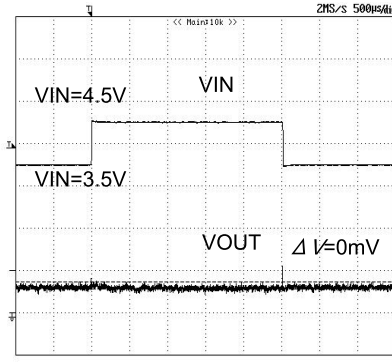
Fig.59 Transient_response (Ta=25°C)
