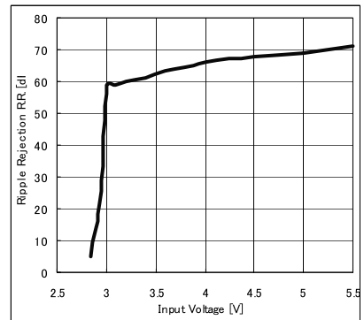
Fig.32 R.R. - VIN
