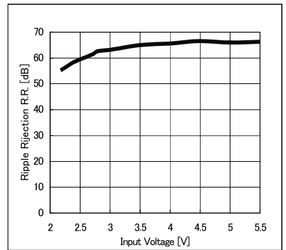
Fig.9 R.R. - VIN
