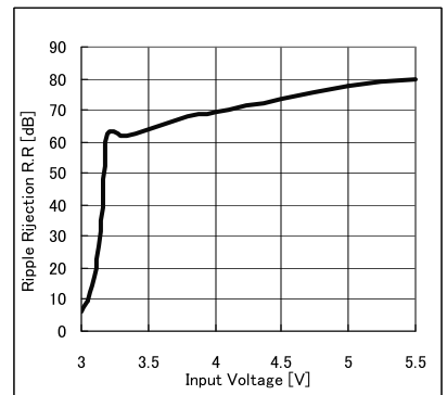
Fig.55 R.R. - VIN
