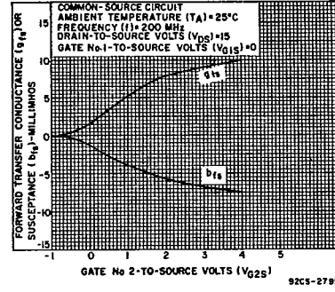
Fig. 6 — Y fs vs. VG2S
