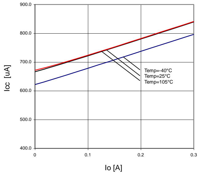
Fig.30 Io-Icc
