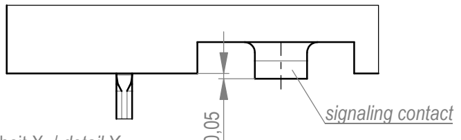
Einzelheit X / detail X M 20:1 / scale 20:1
