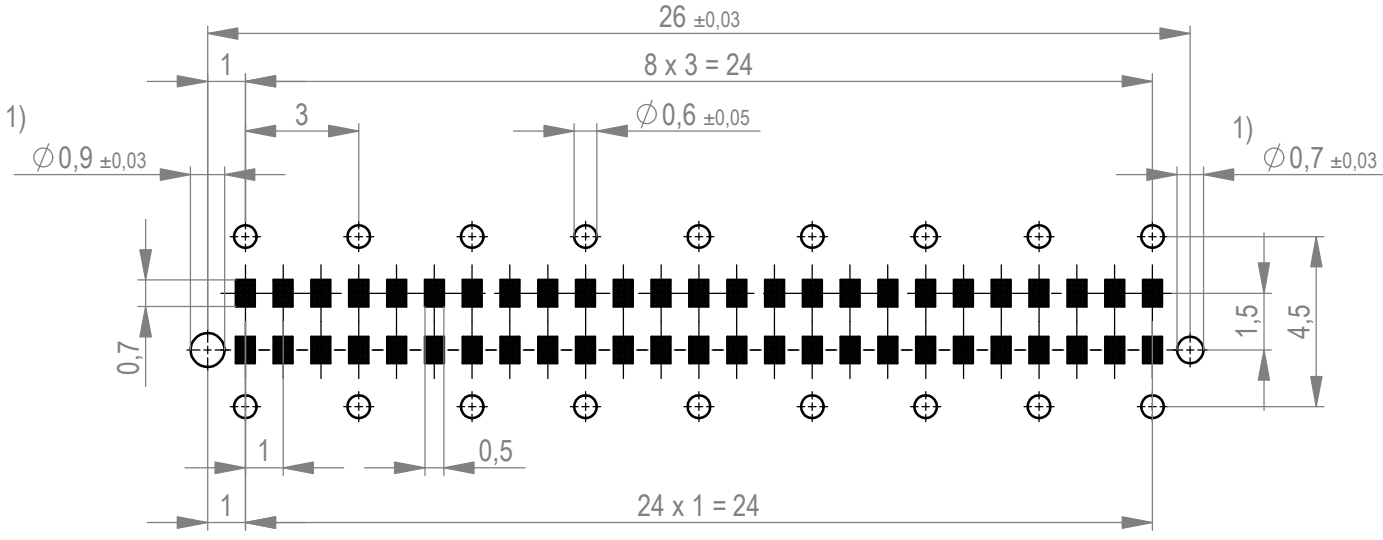
1) Durchmesser des Bohrers / drill tool
