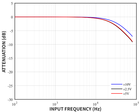
图 36 模拟抗混叠滤波器频率响应
