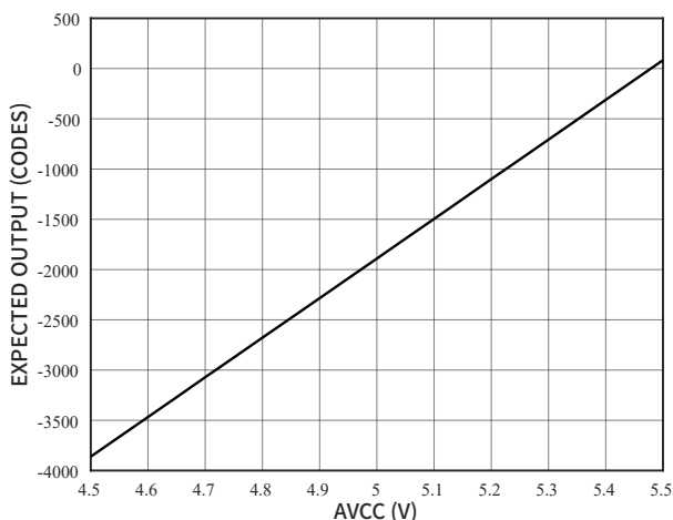
图 47 VCC 诊断传递函数
