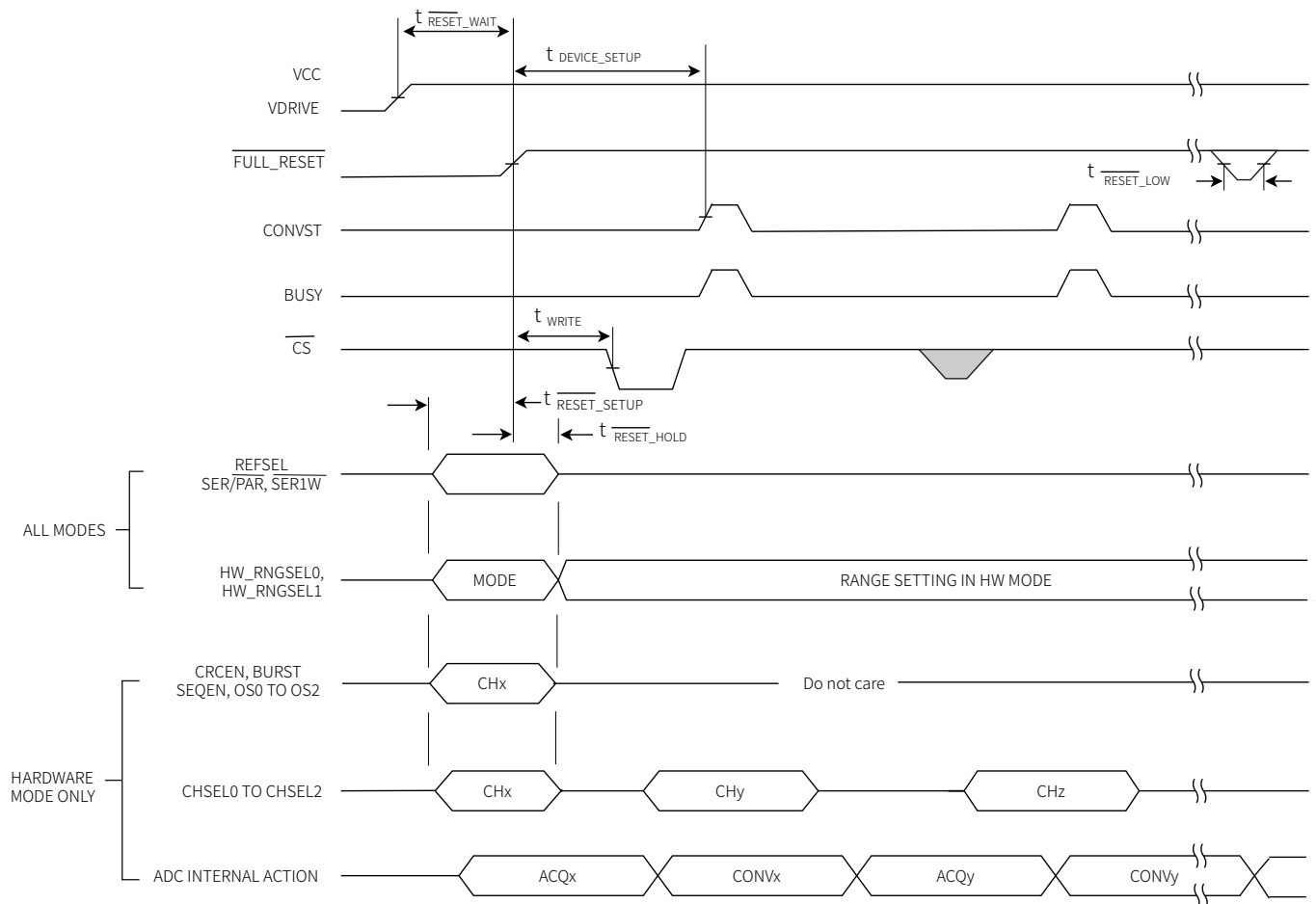
图 3 复位时序图
