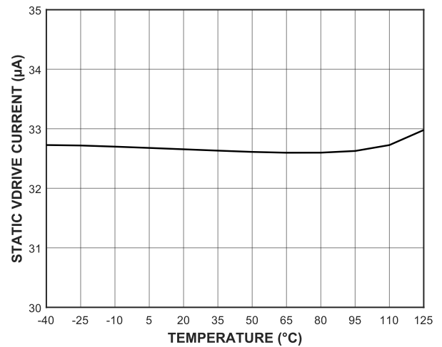
图 29 静态 VDRIVE 电流的温度特性
