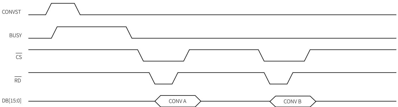
图 50 并行接口转换结果读取
