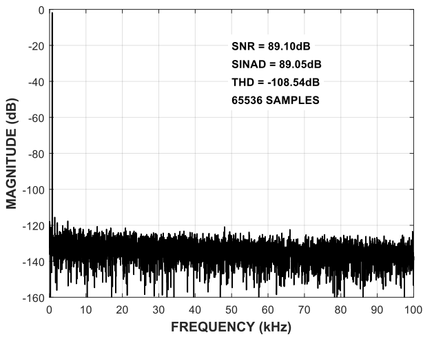
图 16 FFT，±5V 范围
