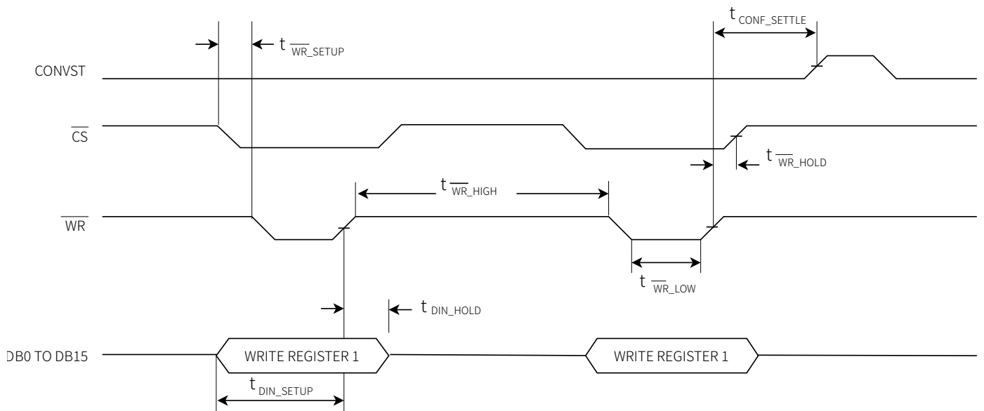
图 6 并行写时序图
