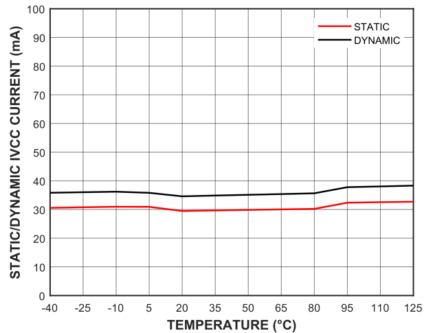
图 31 静态/动态 IVCC 电流的温度特性
