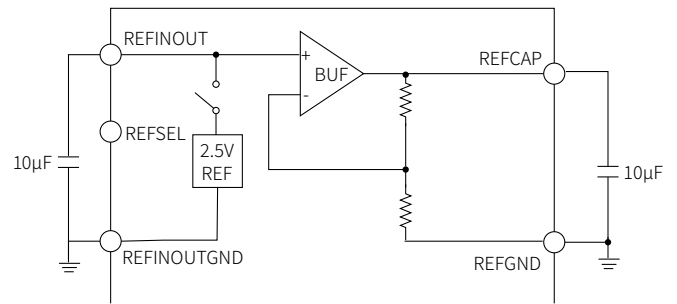
图 37 基准电压电路
