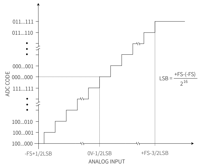
图 38 传递特性
