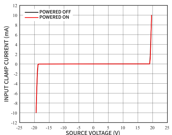
图 34 输入钳位电路 V-I 特性曲线
