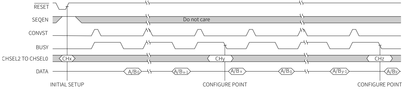
图 43 序列器硬件模式
