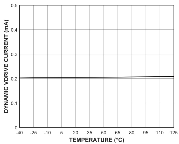
图 32 动态 VDRIVE 电流的温度特性
