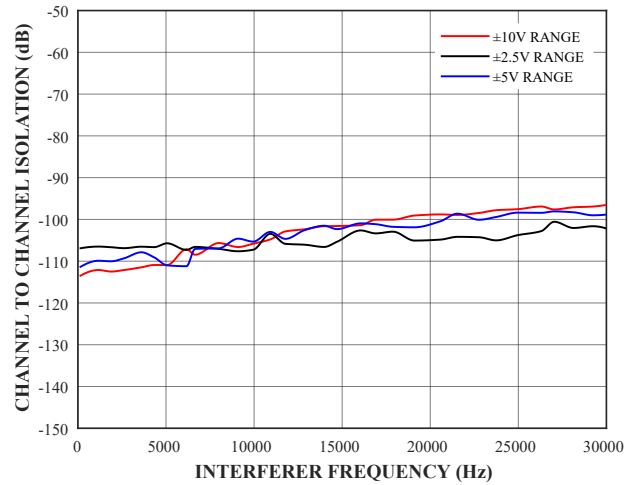
图 27 通道隔离度
