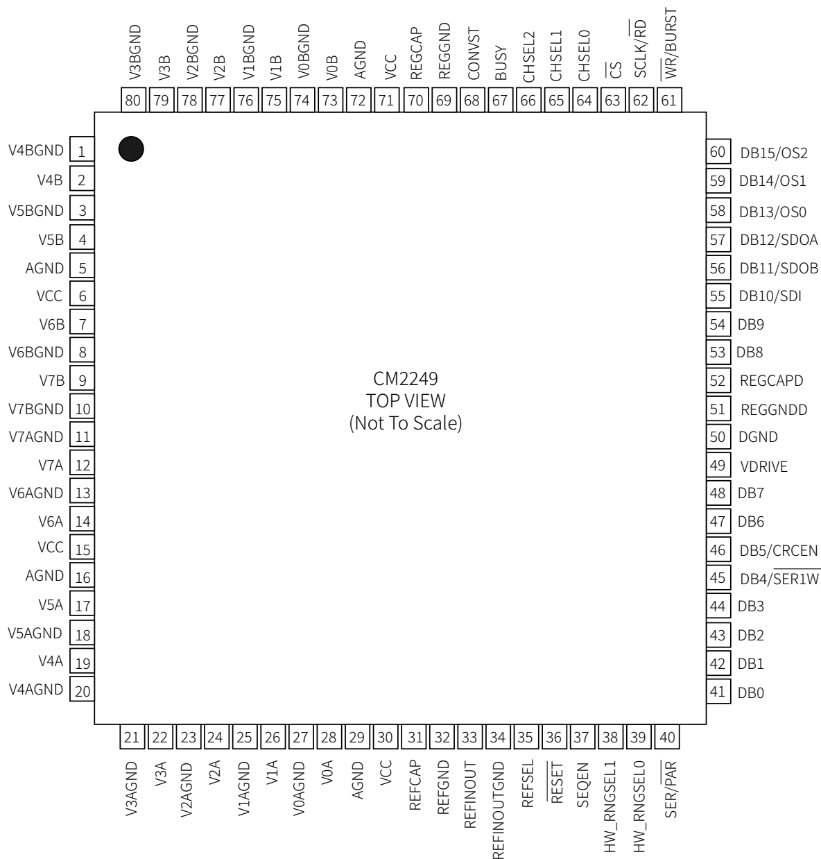
图 1 管脚示意图
