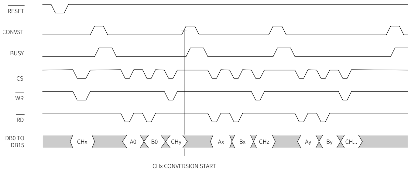
图 42 软件并行模式通道转换设置图
