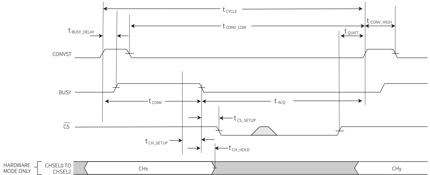
图 2 所有接口的通用时序图
