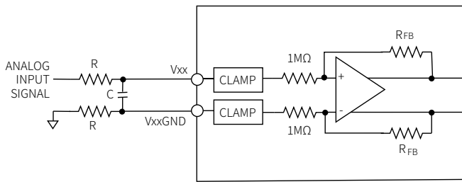
图 35 模拟输入电阻匹配
