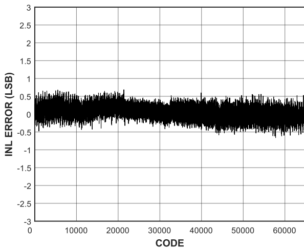
图 8 典型 INL 误差, ±10V 范围
