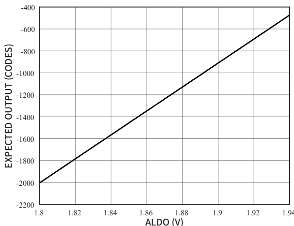
图 48 ALDO 诊断传递函数
