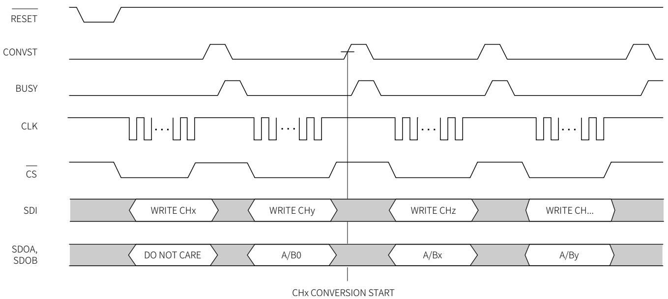
图 41 软件串行模式通道转换设置图
