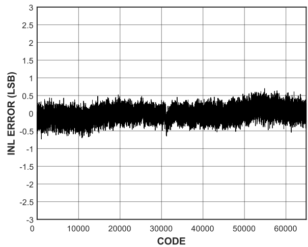
图 9 典型 INL 误差, ±5V 范围
