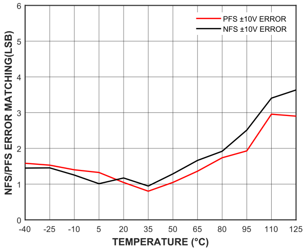
图 26 PFS/NFS 误差匹配的温度特性, ±10V 范围
