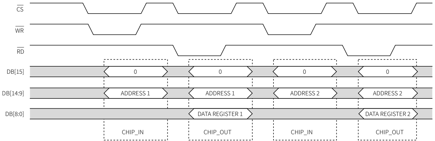
图 52 并行接口寄存器读操作
