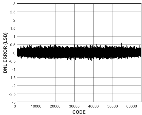
图 11 典型 DNL 误差, ±5V 范围
