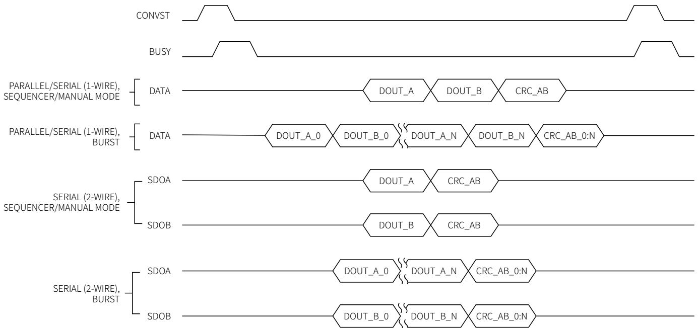
图 49 所有模式的 CRC 回读
