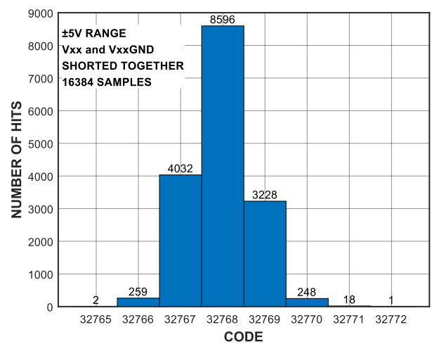
图 13 零输入直方图, ±5V 范围
