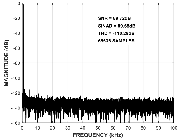
图 15 FFT，±10V 范围
