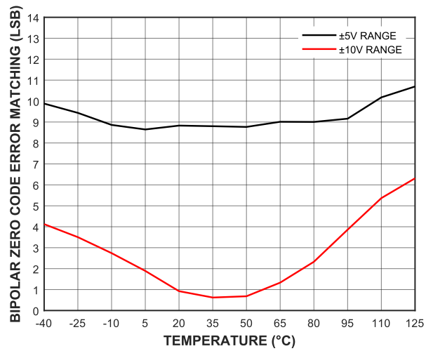
图 23 双极性零误差匹配的温度特性
