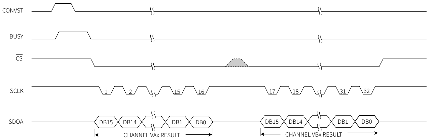
图 54 1 线串口模式转换结果读取
