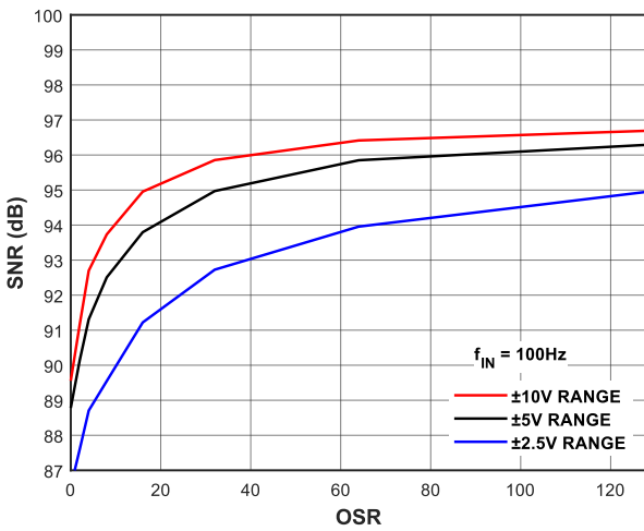
图 28 不同过采样率下 SNR 与 OSR 的关系
