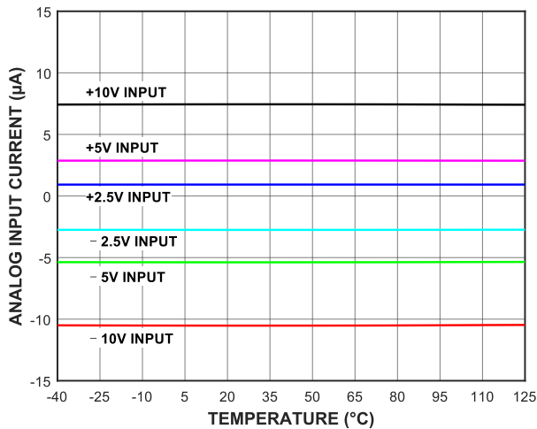
图 30 不同电源电压下模拟输入电流的温度特性
