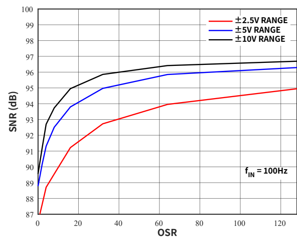
图 39 SNR 与 OSR 的关系图
