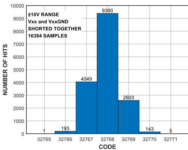
图 12 零输入直方图, ±10V 范围
