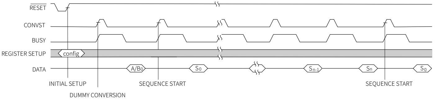
图 44 序列器软件模式
