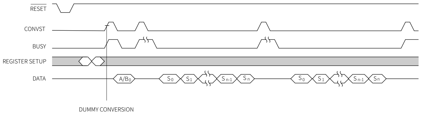
图 46 突发序列器软件模式
