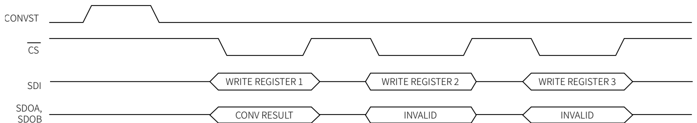
图 55 串行接口寄存器写操作
