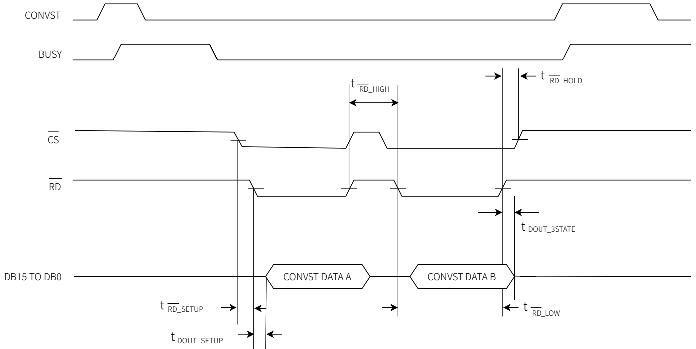
图 5 并行读时序图
