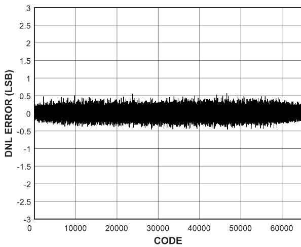
图 10 典型 DNL 误差, ±10V 范围
