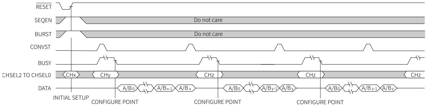
图 45 突发序列器硬件模式
