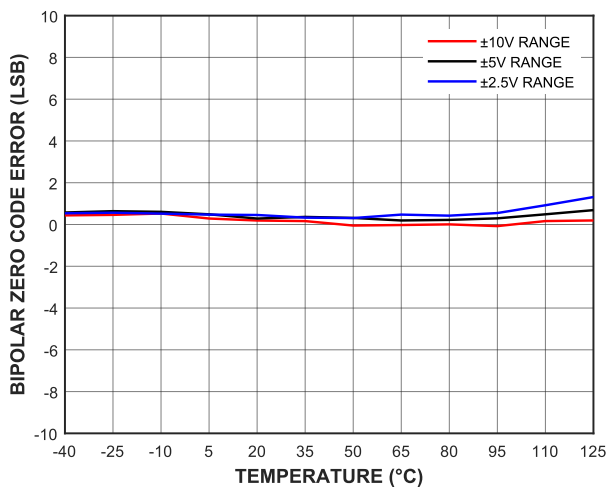
图 22 双极性零代码误差的温度特性
