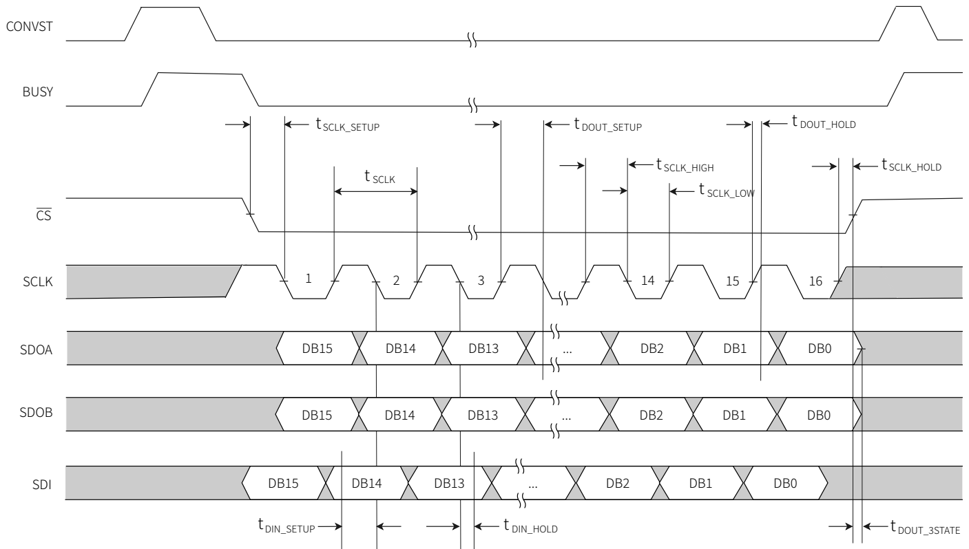
图 7 串行时序图
