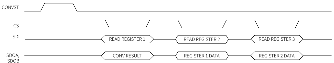
图 56 串行接口寄存器读操作
