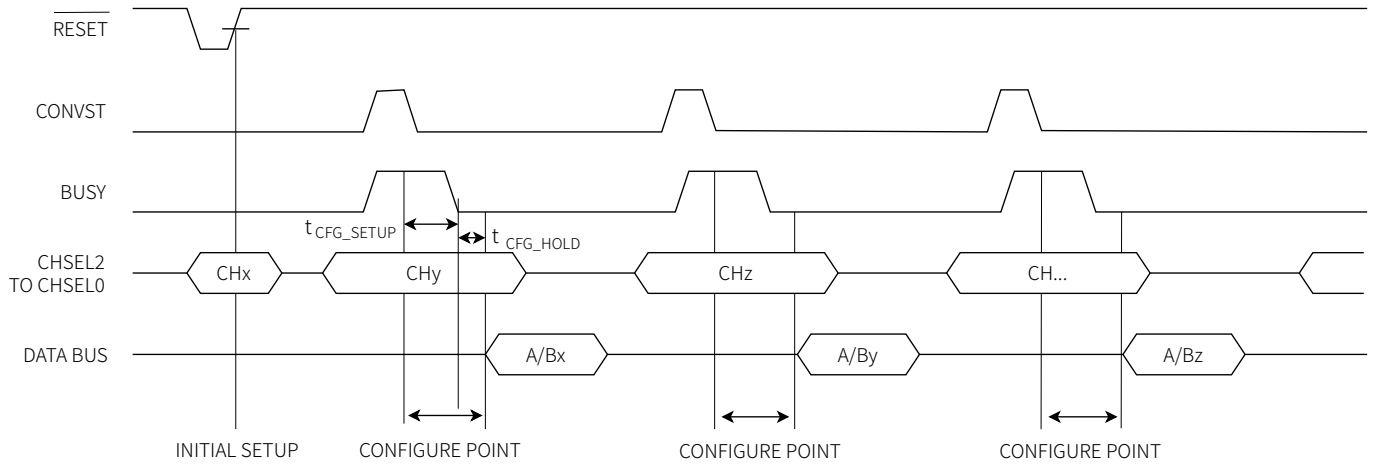
图 40 硬件模式通道转换设置图
