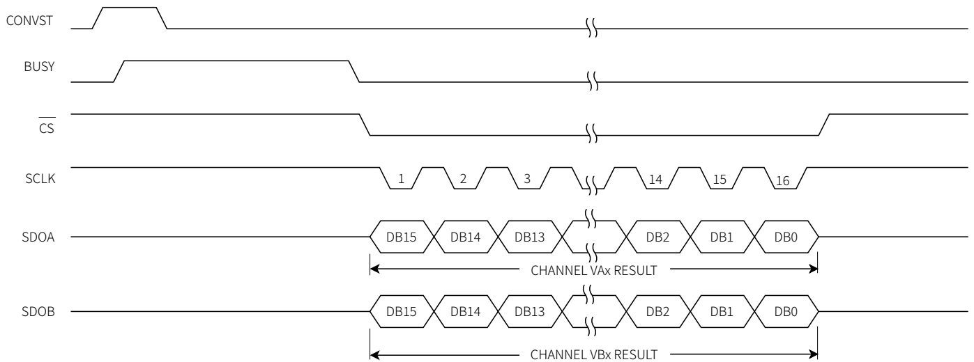
图 53 2 线串口模式转换结果读取
