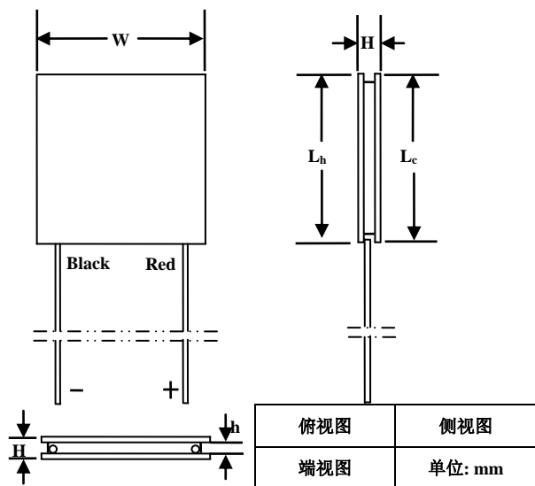
图 10. 密封ATE1-71的机械尺寸
