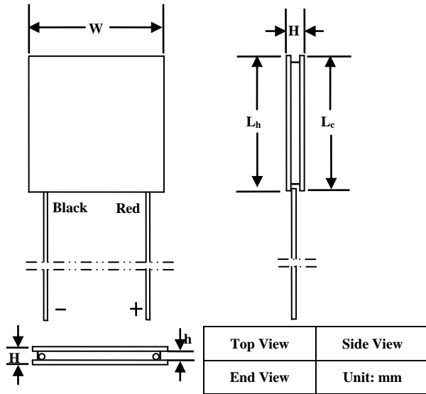
图 10. 密封ATE1-127的机械尺寸
