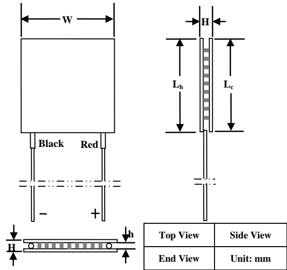
图11. 非密封ATE1-127的机械尺寸
