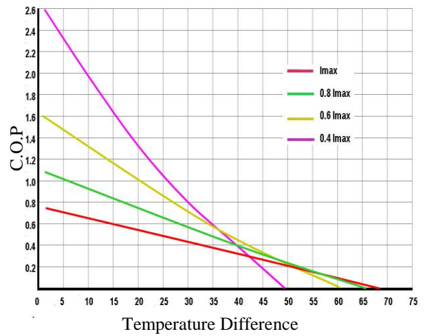
图 9. C.O.P 与 DT 的关系图
