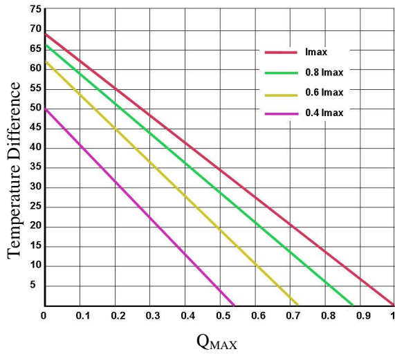
图 6. DT 与 Q_{MAX} 的关系图
