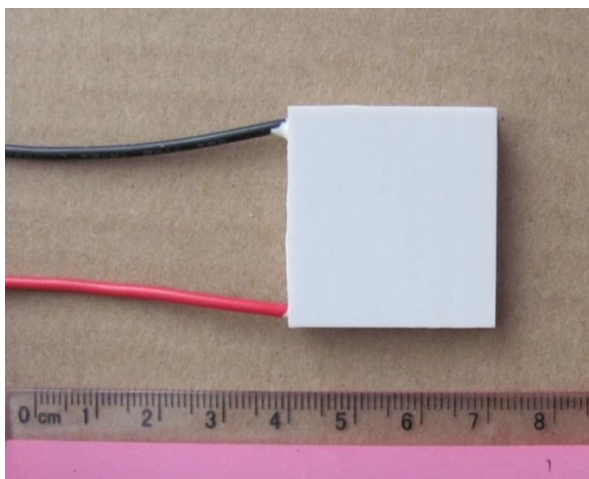
图 1.1 ATE1-127 的实体照片
