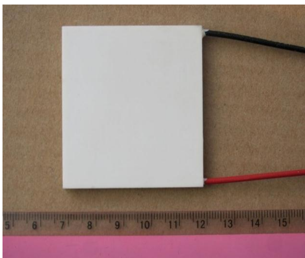
图 1.3 ATE1-127 的实物侧面图
