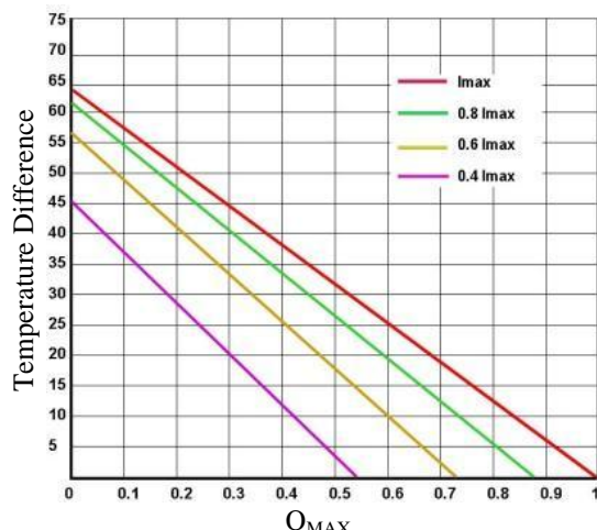
图 2. DT 与 Q_{MAX} 的关系图
