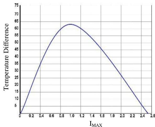
图3. DT与 I_{MAX} 的关系图
