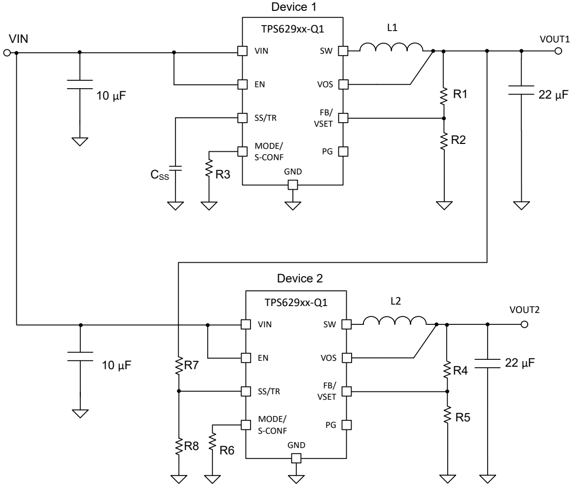
图 9-83. Tracking Example
