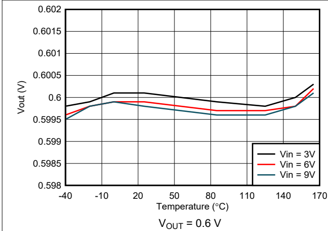
图 7-9. Output Voltage Accuracy - VSET Selected
