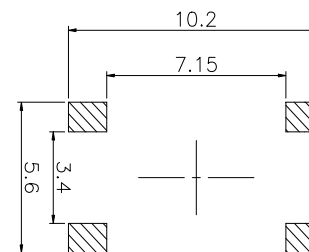
PCB. 焊接图
