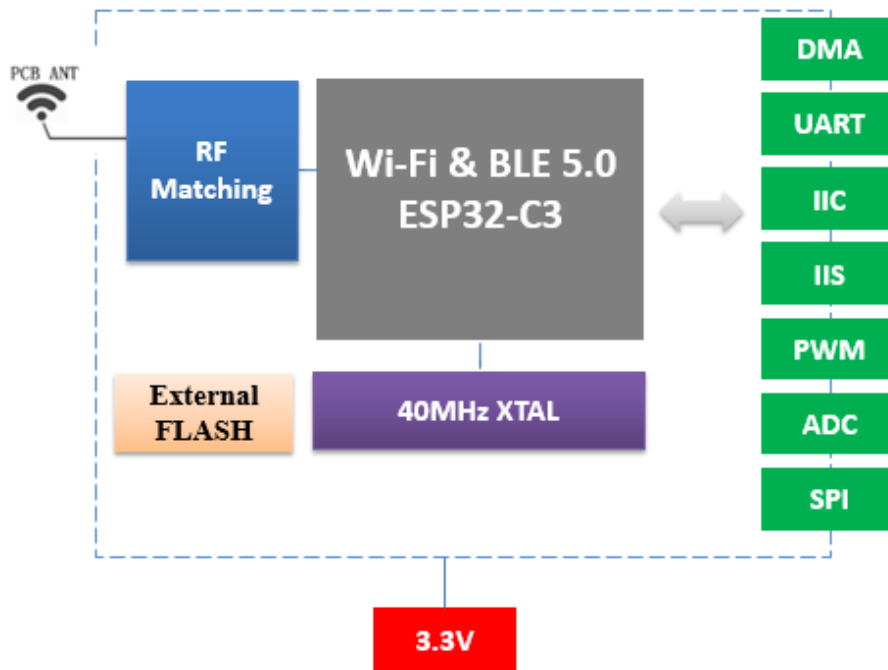
Fig.1.1 ESPC3-12E Module Structure
