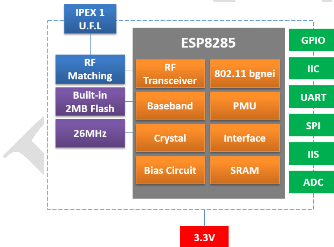
Fig. 1.1 ESP-M1 Module Structure
