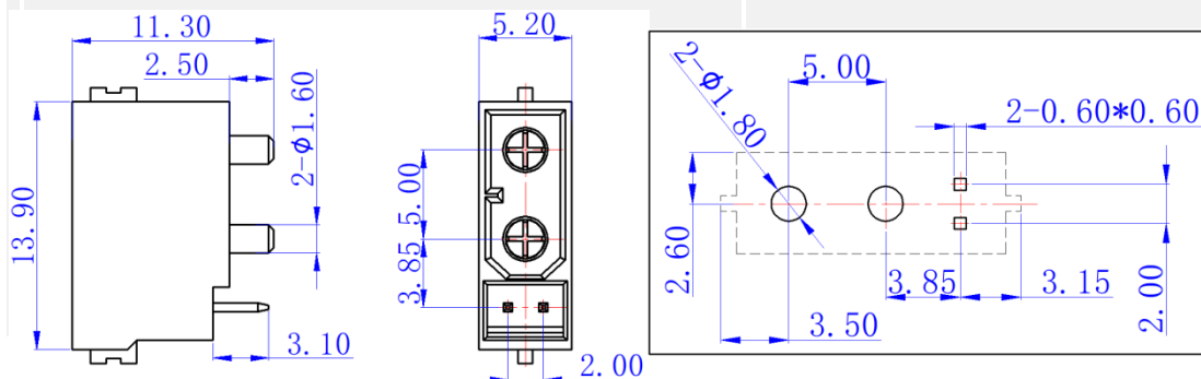
安装孔尺寸示意图
