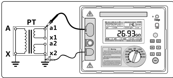
图 22 (二次绕组间绝缘电阻测试)
