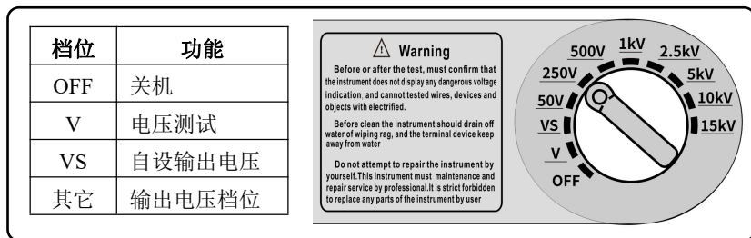
图 2 （旋钮档位图）
