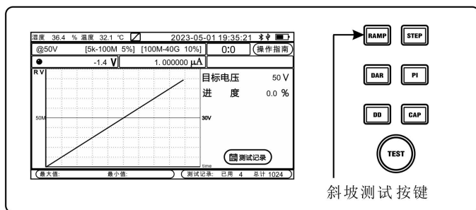
图 8 (斜坡 RAMP 测量)
