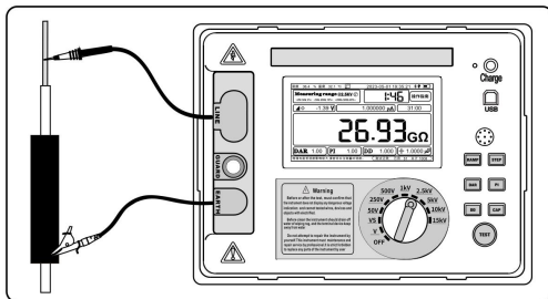
图 16（接常规两线测量接线方式）
