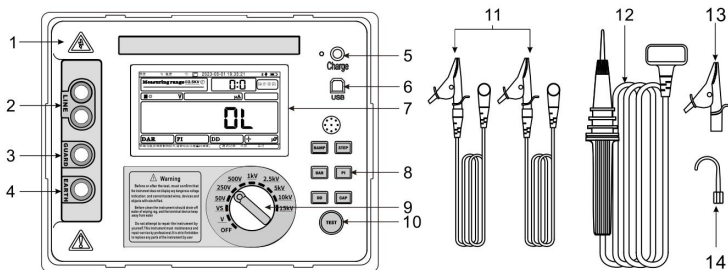
图 1（仪表结构图）
