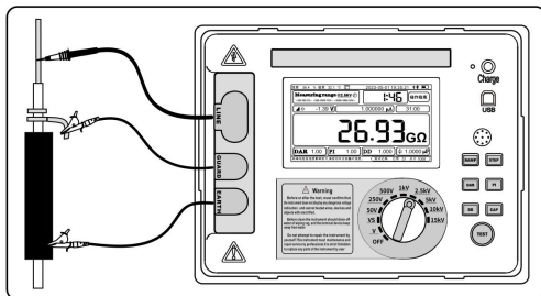
图 17（超高阻值三线测量接线方式）
