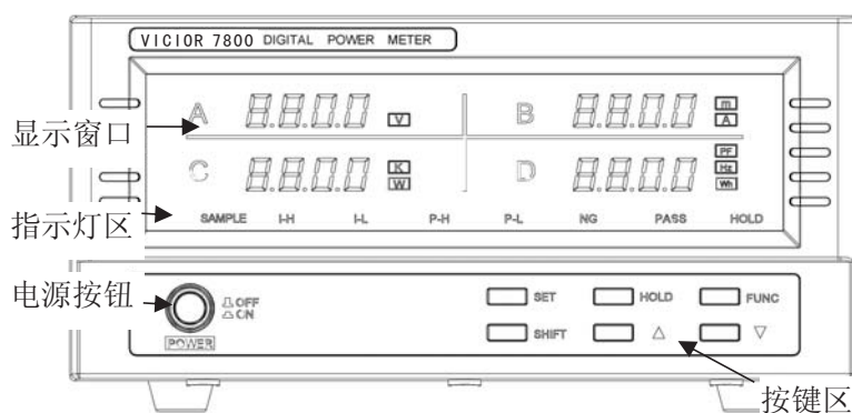
图 1 前面板
