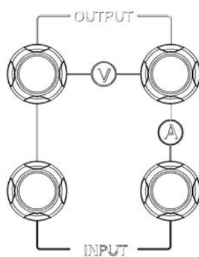
图 3 接线图
