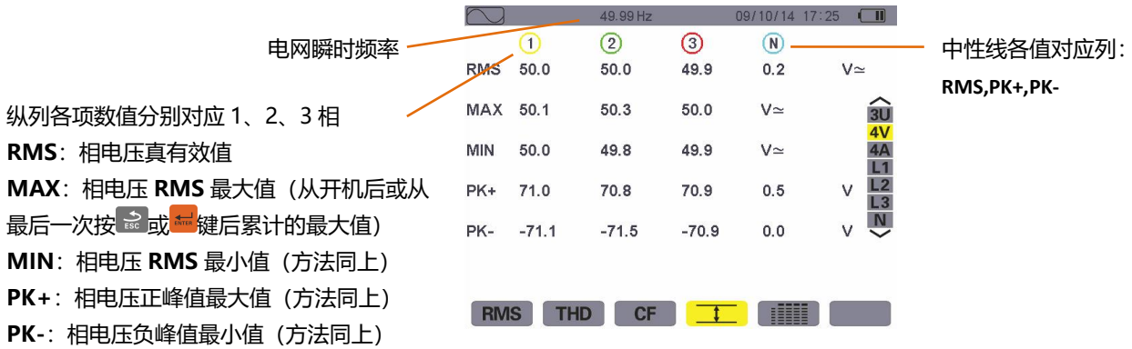
图 8-13 4V 下 Max.-Min.显示屏幕
