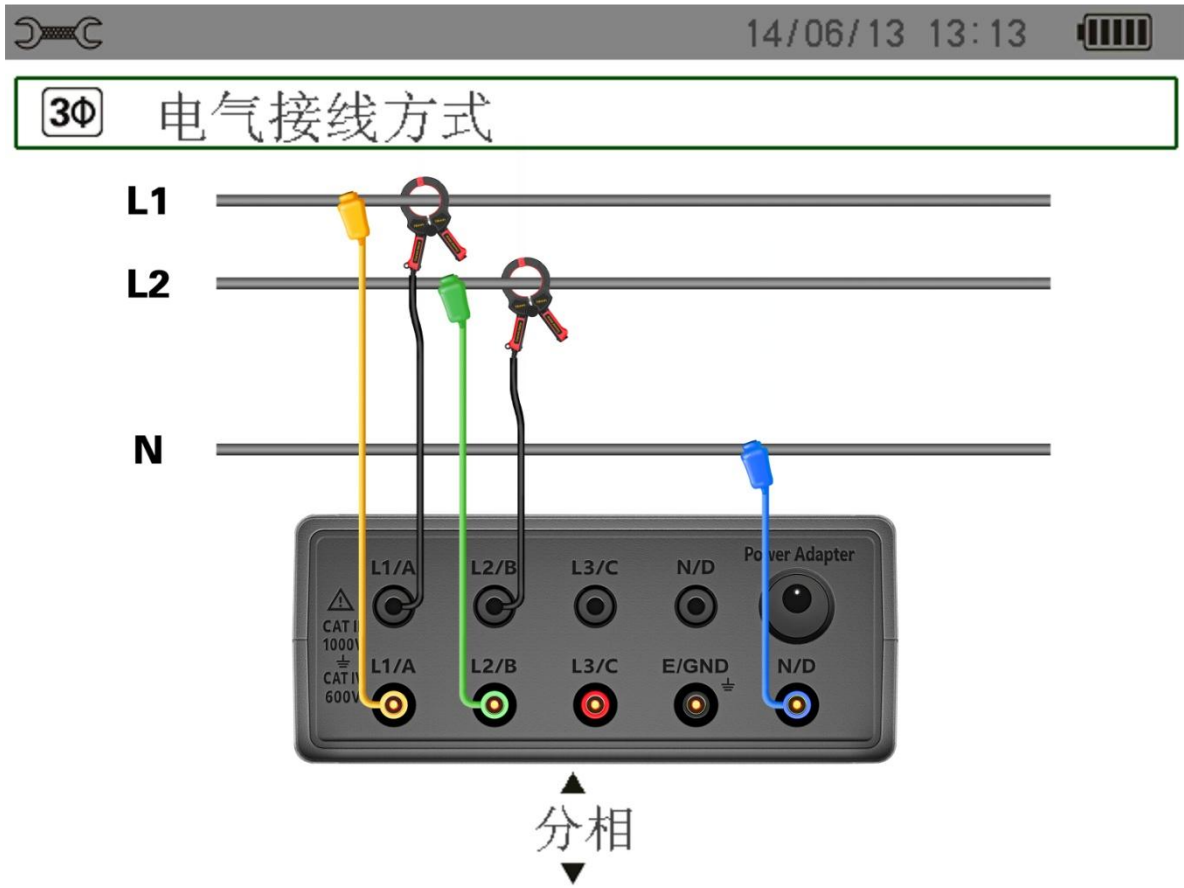
图 4-5 分相连接
