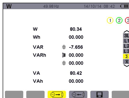
图 11-6 电能消耗三相总和显示屏幕
