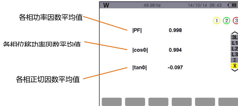
图 11-7 三相算术平均数显示屏幕
