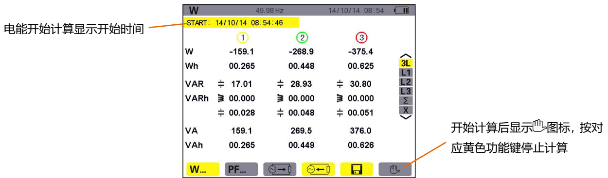
图 11-10 开始电能计算时的功率和电能显示屏幕
