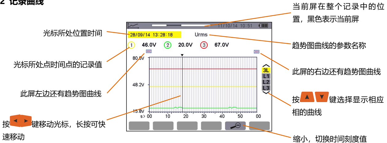
图 10-10 线电压有效值不包括最大、最小、平均值
