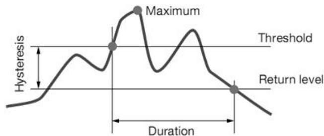
图 18-1 骤升侦测回差图例
