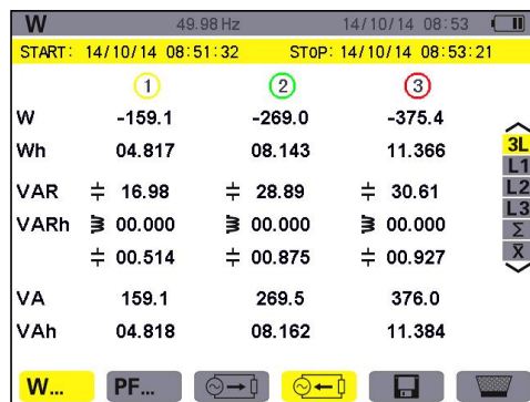
图 11-8 三相(3L)电能产生显示屏幕
