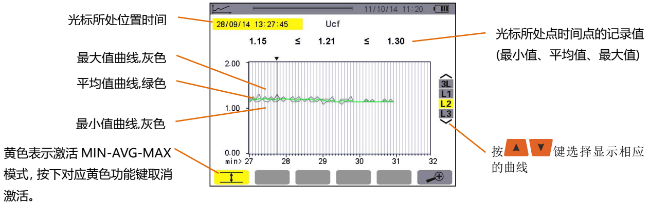
图 10-13 L2 的 Ucf 包括最大、最小、平均值
