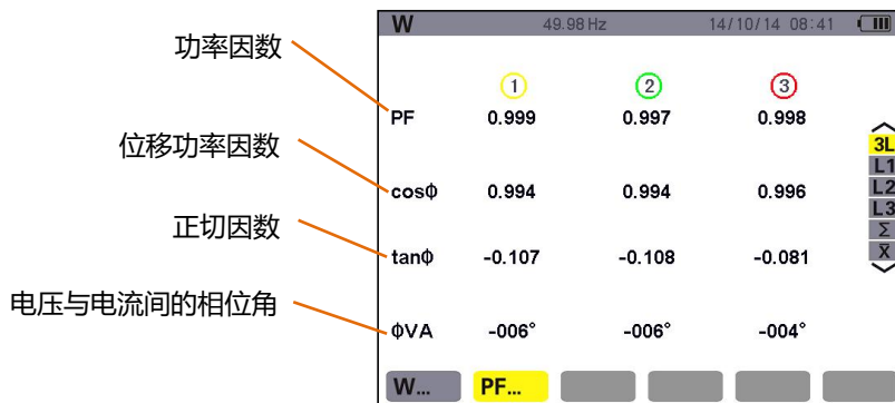
图 11-5 三相(3L)功率因数屏幕显示
