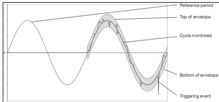
图 18-4 暂态捕捉触发原理解
