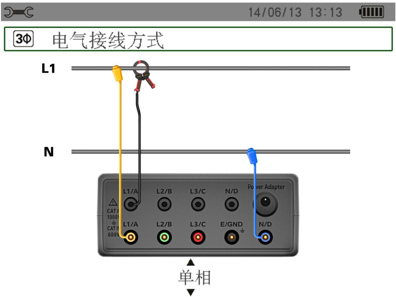
图 4-4 单相连接
