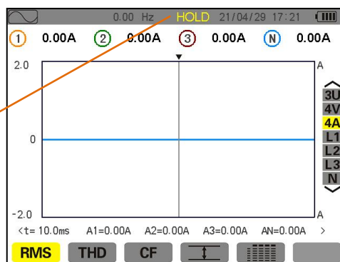
图 16-2 WAVE 模式下的 HOLD 界面
