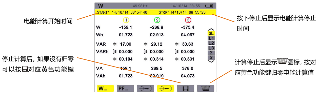
图 11-11 停止电能计量时的功率和电能模式屏幕
