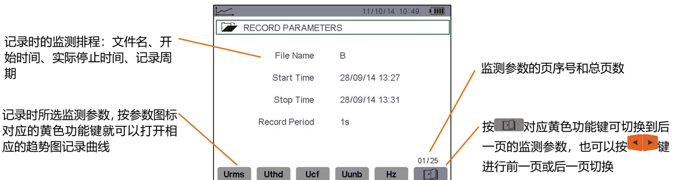
图 10-9 趋势图记录列表子菜单显示
