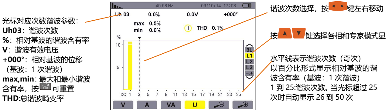
图 7-9 线电压谐波 L1 显示
