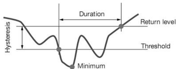
图 18-2 骤降侦测回差图例
