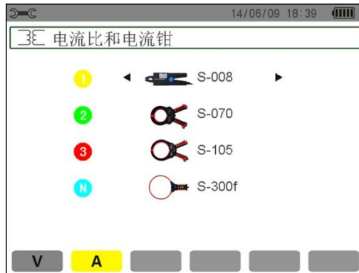
图 5-8 电流钳及变比设置菜单
