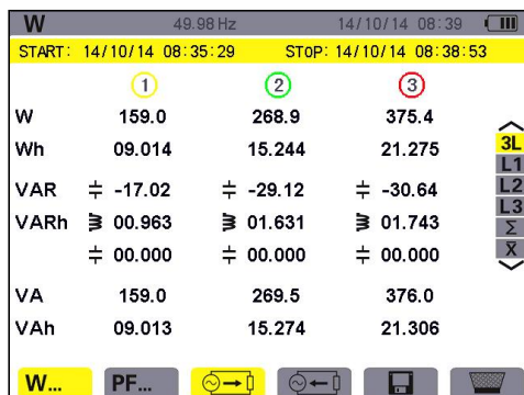
图 11-3 三相(3L)消耗电能的屏幕显示
