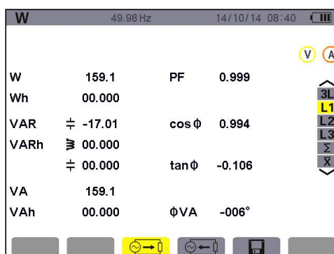
图 11-4 L1 相电能消耗显示屏幕
