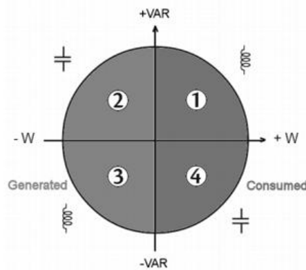
图 18-3 功率电能象限图
