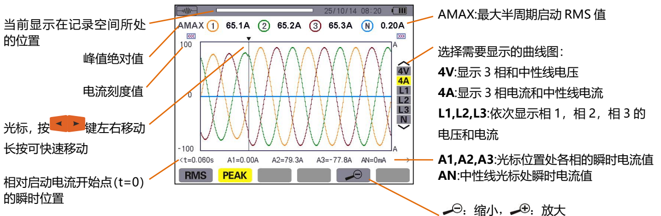
图 6-11 4A 峰值显示屏幕
