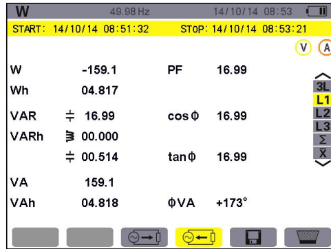
图 11-9 L1 相电能产生显示屏幕
