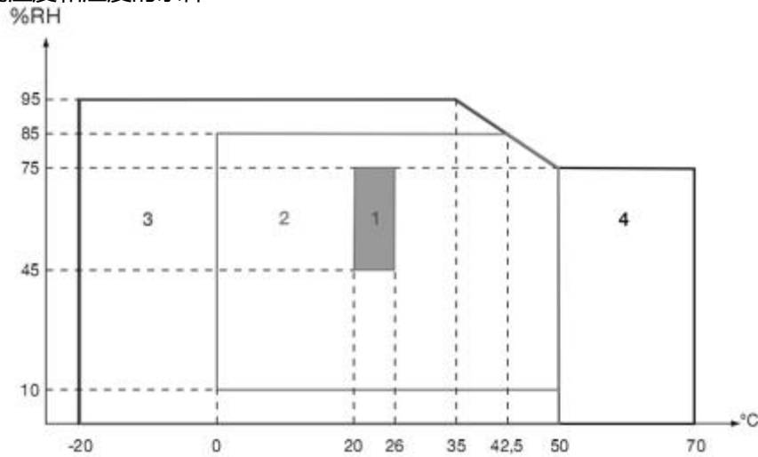
图 19-1 温湿度条件图示
