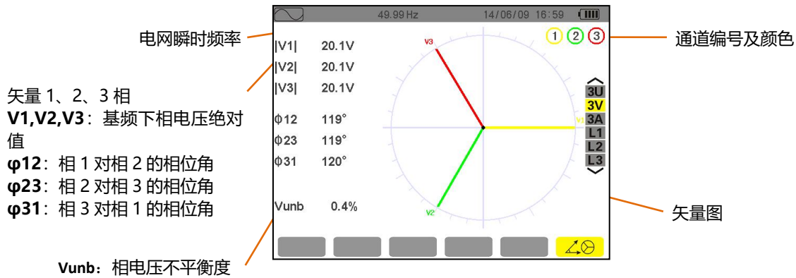
图 13-1 3V 下矢量图显示屏幕
