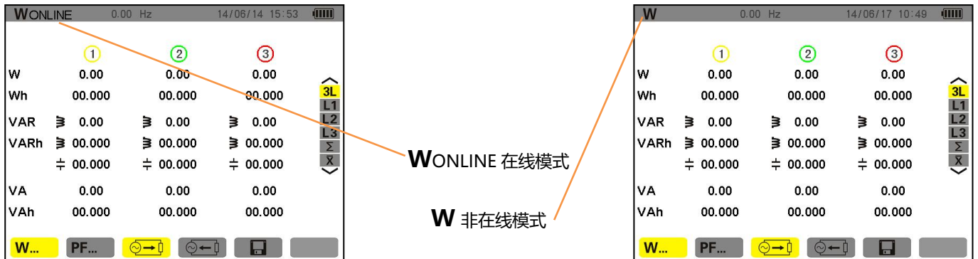
图 11-1 两种模式下的界面区别
