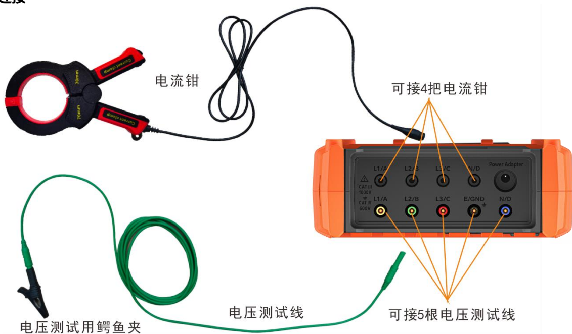
图 4-3 顶端测试连接
