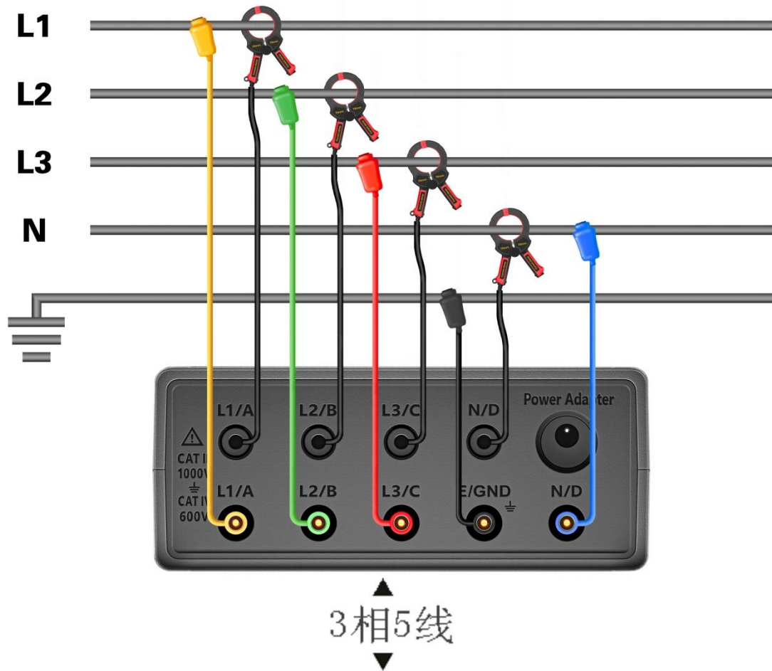
图 4-7 三相 5 线连接
