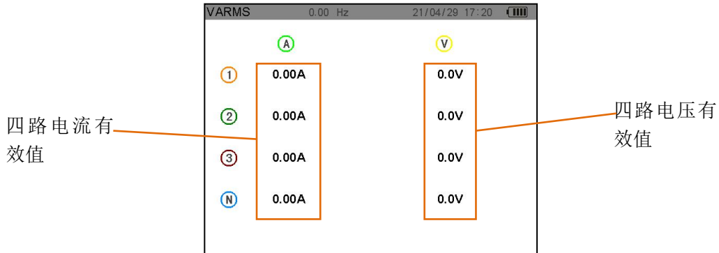
图 14-1 电流电压有效值界面
