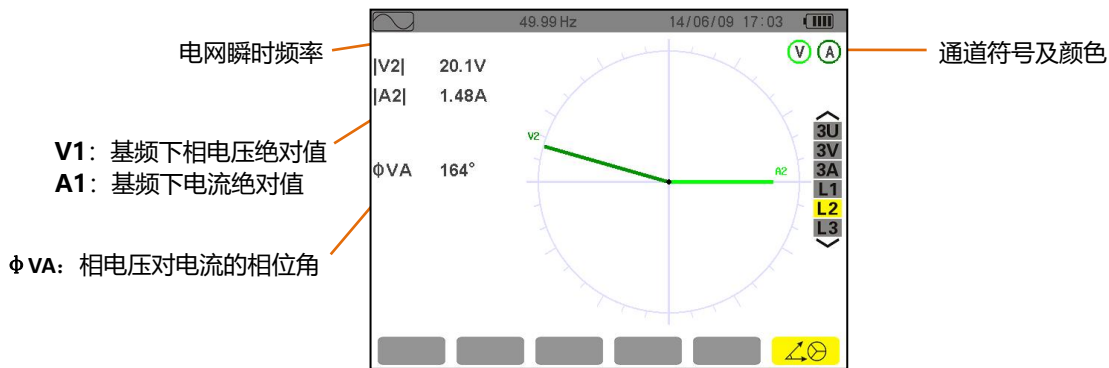
图 13-2 L1 下矢量图显示屏幕
