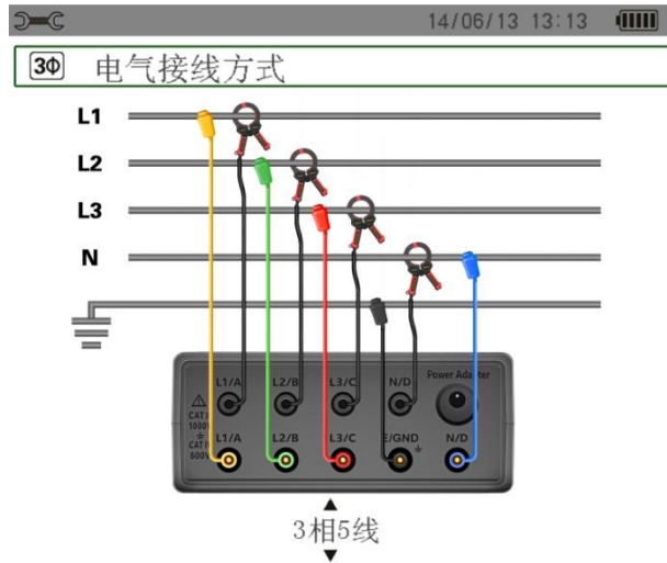
图 5-6 电气连接方式选择
