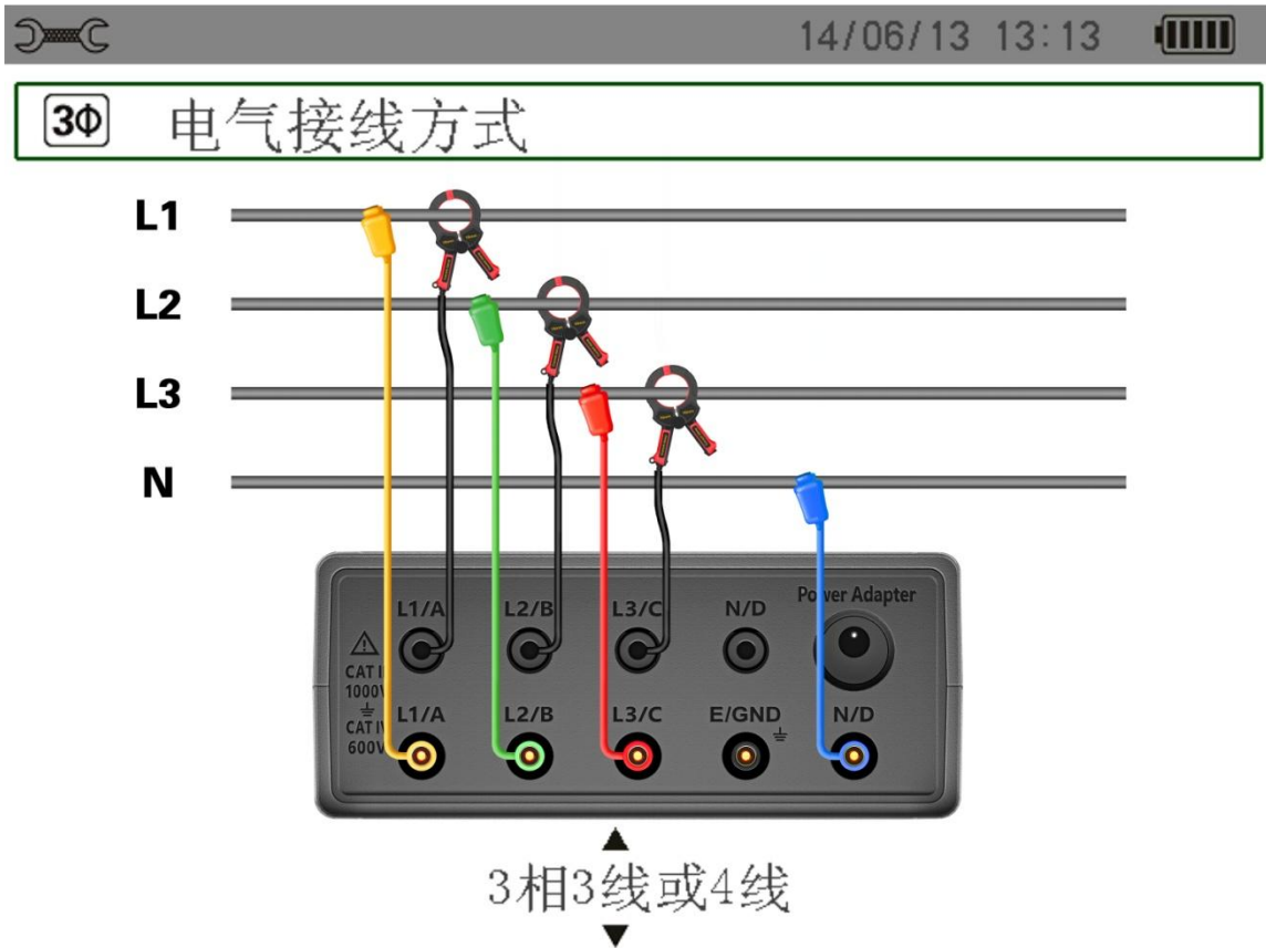
图 4-6 三相 3 线或 4 线连接
