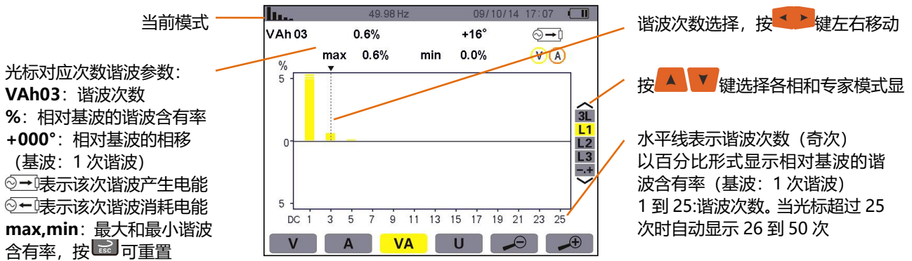
图 7-7 视在功率谐波 L1 显示
