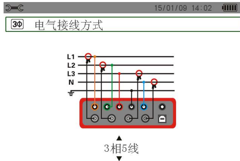
图 4-7 三相5线连接
