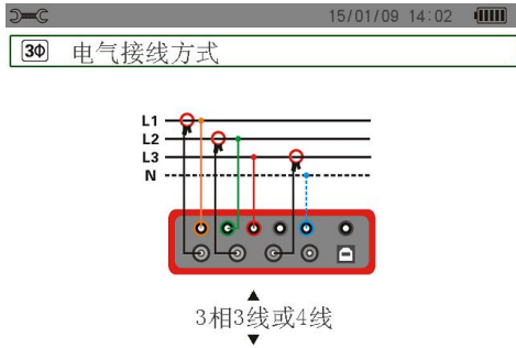
图 4-6-1 三相4线
