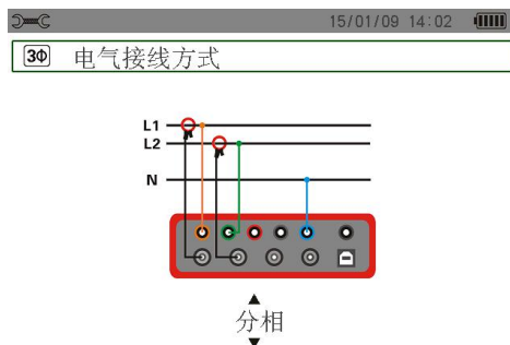
图 4-5 分相连接
