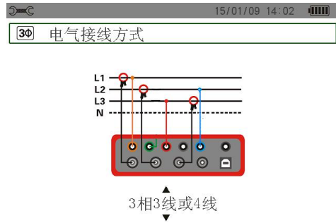
图 4-6-2 三相3线
