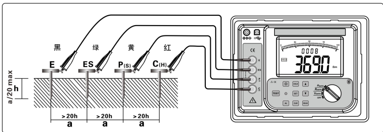
图 8 (土壤电阻率测试示意图)
