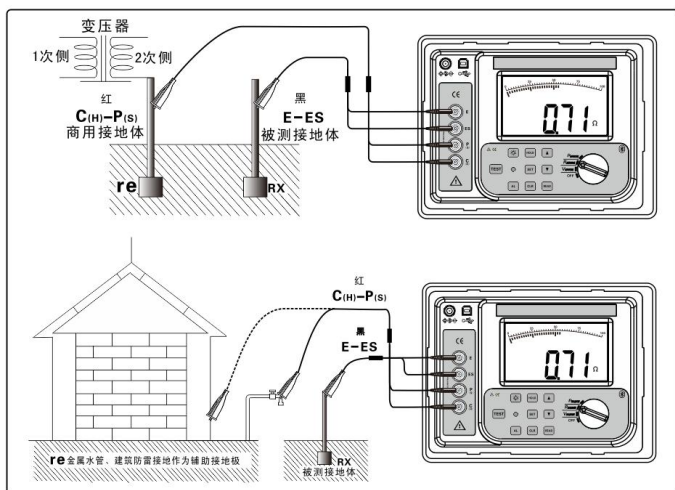
图 7（二线测试接地电阻示意图）
