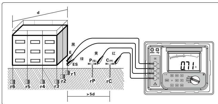
图 4（四线精密测试接地电阻示意图）
