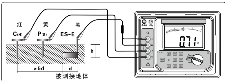
图 6（三线测试接地电阻示意图）
