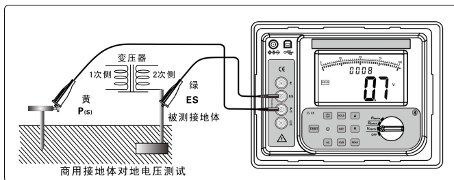
图 10（接地电压测试示意图）
