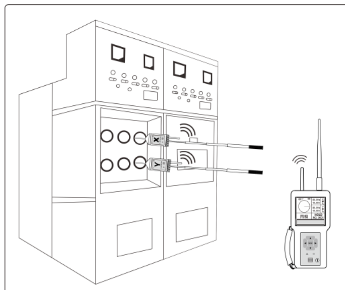
中置柜普通核相（使用探针和绝缘杆）
