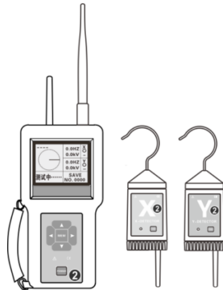
2号核相仪（普通核相）
