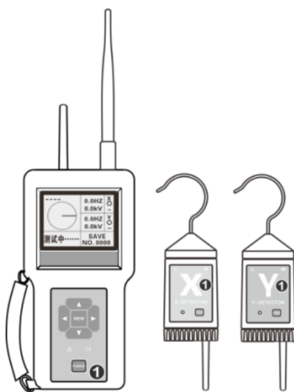
1号核相仪（普通核相）
