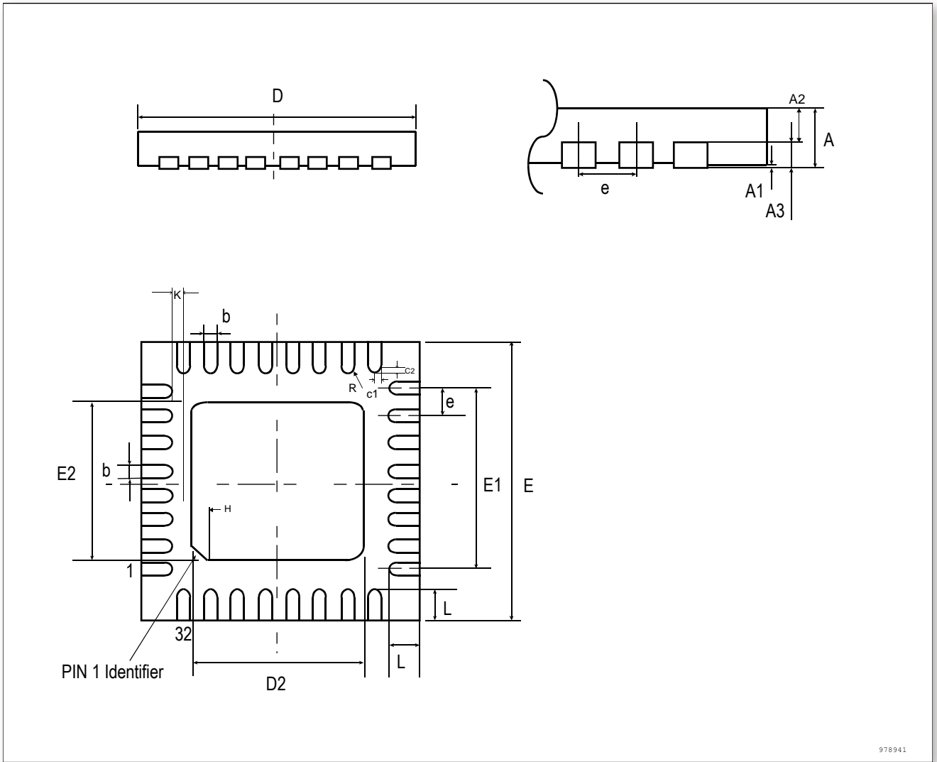
图 19 QFN32, 32 脚方形扁平无引线封装外形封装图
