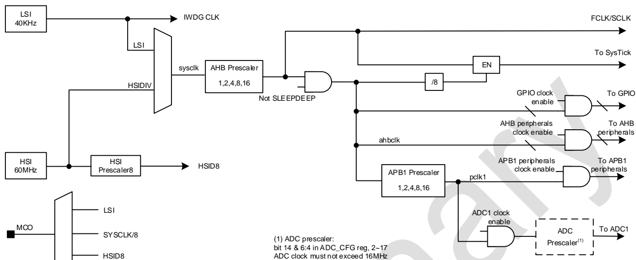
图 4 时钟树
