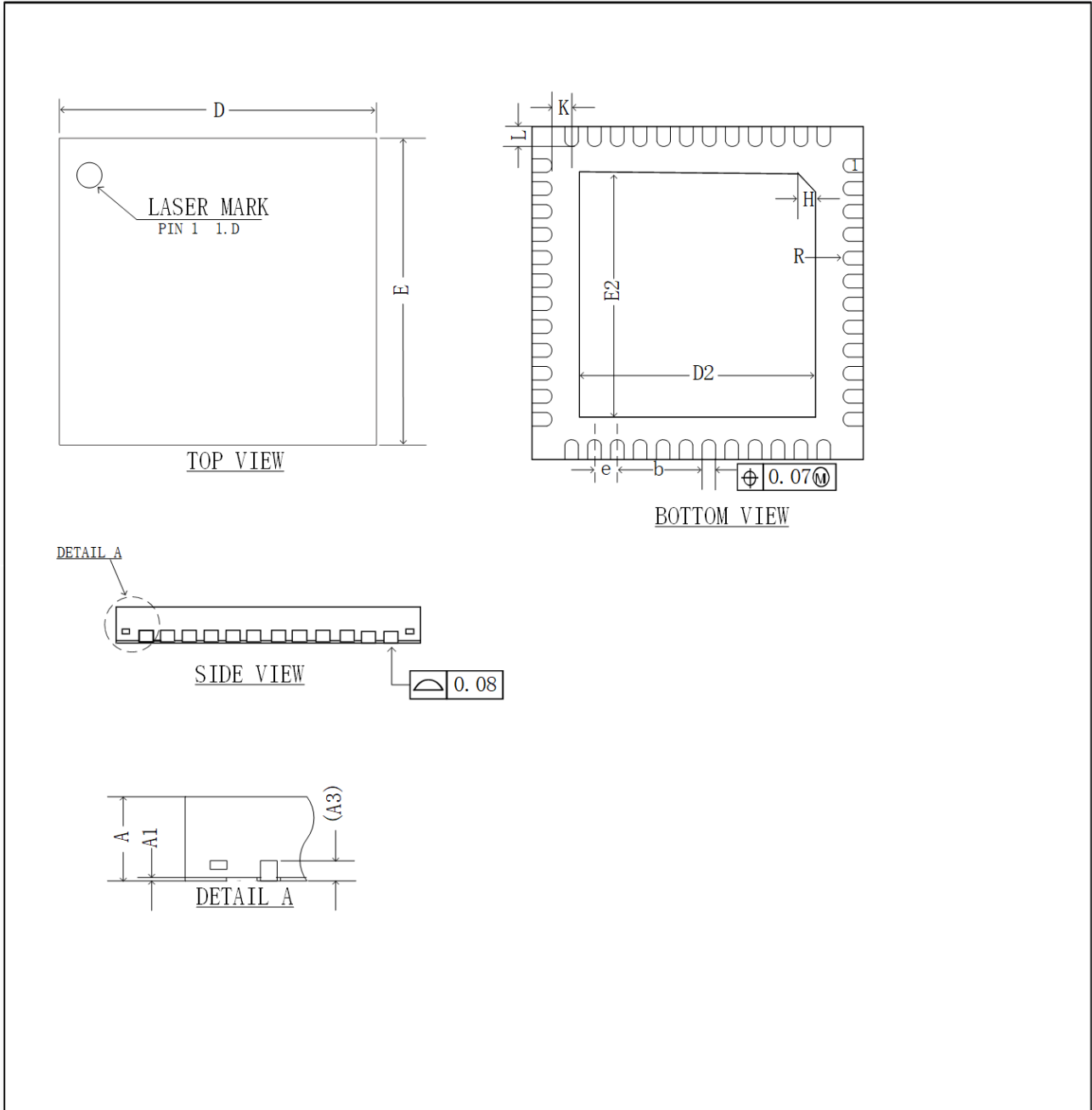
图 18 QFN48 脚底剖面方形扁平封装图
