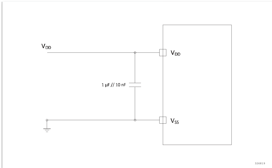
图 16 供电电源和参考电源去耦线路
