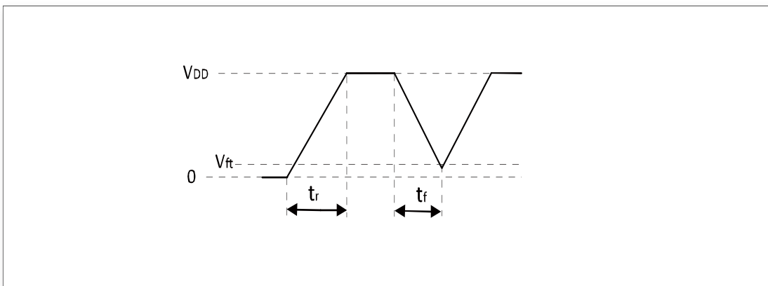
图 11 上电与掉电波形
