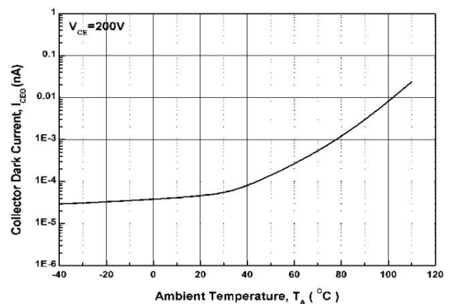
图6 暗电流与环境温度的关系 Fig.6 Dark Current vs Ambient Temperature
