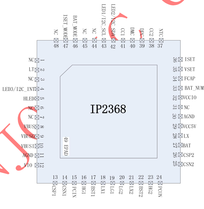
图 2 IP2368 引脚图
