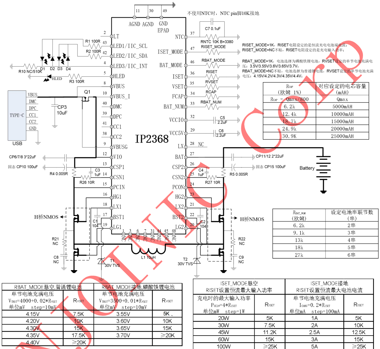
图 13 应用原理图
