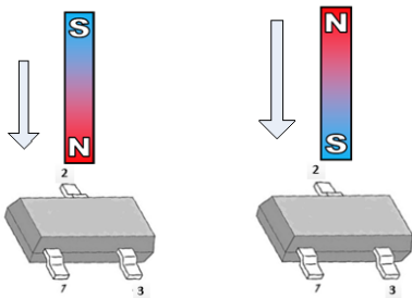
VOUT=低电平
