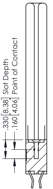
SECTION A-A
