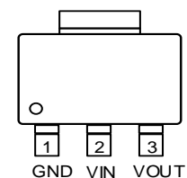
SOT-89-3 ( R-Type )
