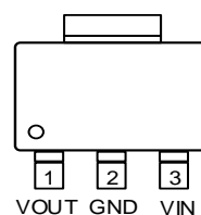
SOT-89-3 ( L-Type )
