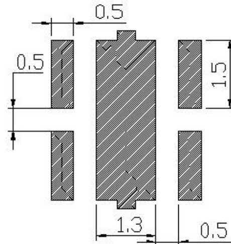
焊盘建议图
