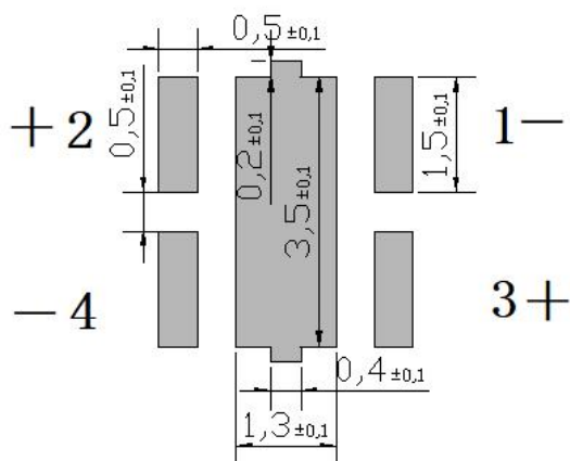
焊盘建议大小
