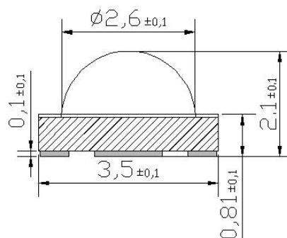
侧面图 120°
