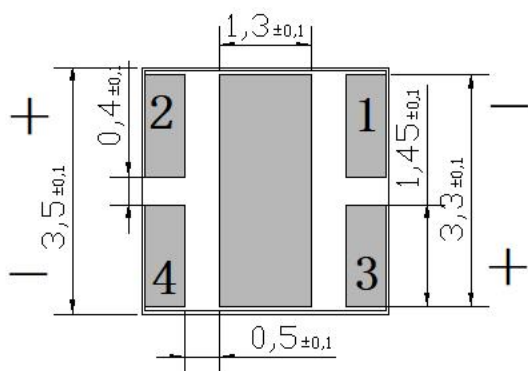
焊盘建议大小
