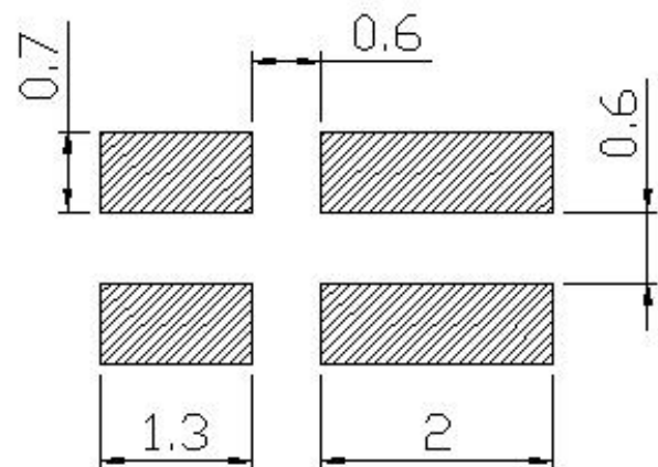
焊盘建议图
