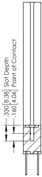
SECTION A-A
