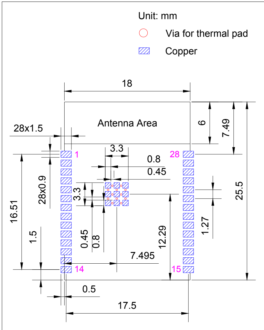
图 7: 推荐 PCB 封装图形
