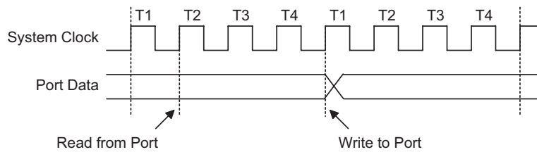
读写时序
