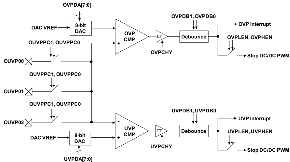
过压 / 欠压保护方框图
