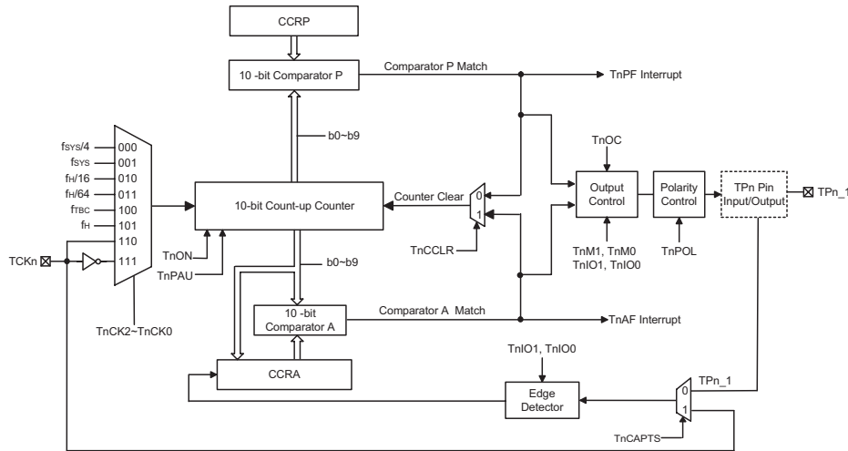
周期型 TM 方框图 (n=1) – HT45FH4MA/HT45FH4MA-1
