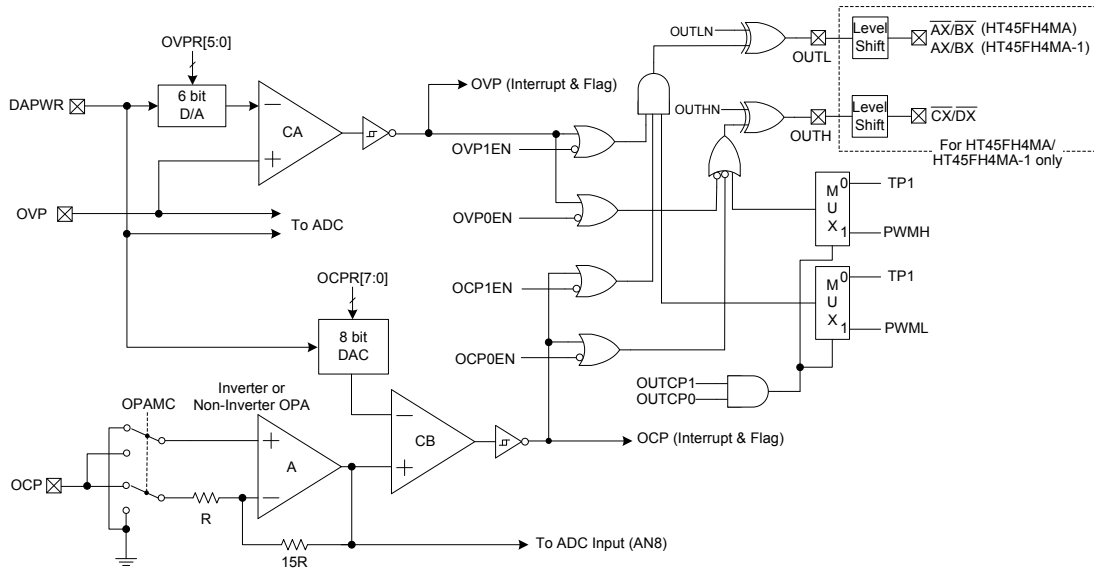
过电压 / 过电流保护方框图
