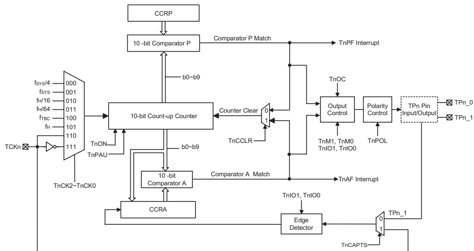
周期型 TM 方框图 (n=1) – HT45F4MA
