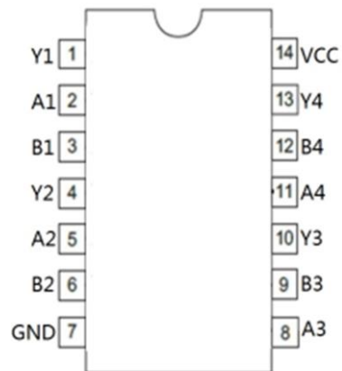
DIP14/SOP14
