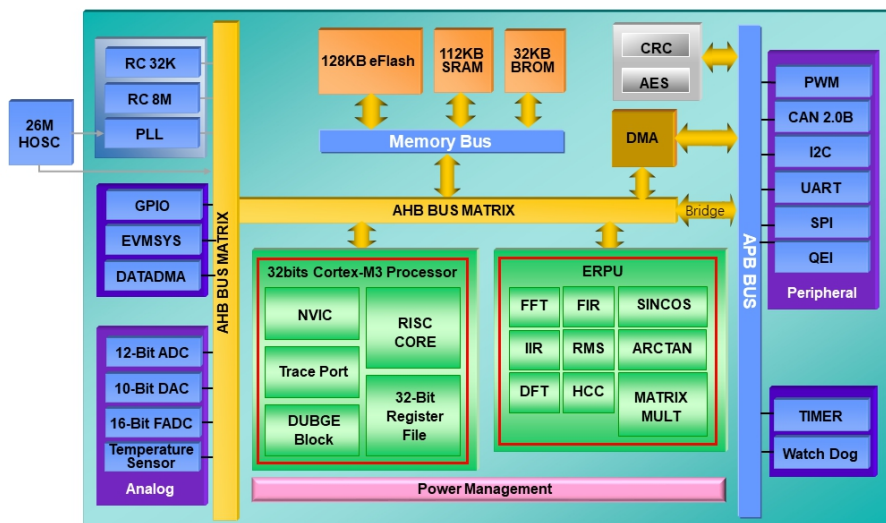
图 2-1 TMF6200 的系统框图
