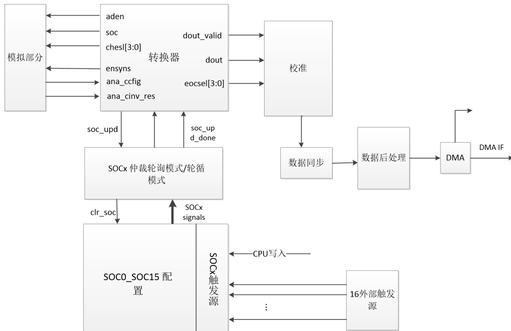
图 8-3 FSARADC 模块框图
