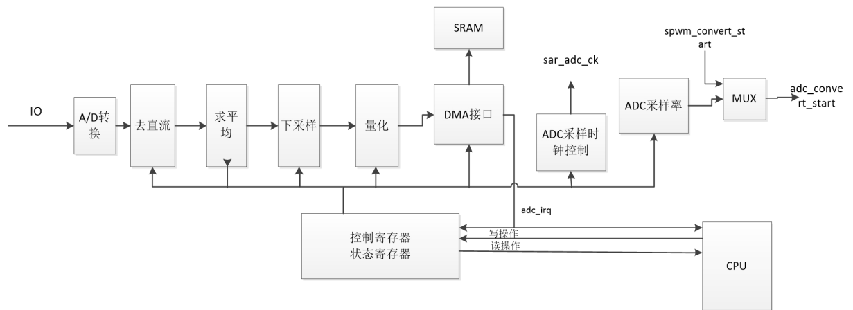
图 8-1 SARADC0~13 框图
