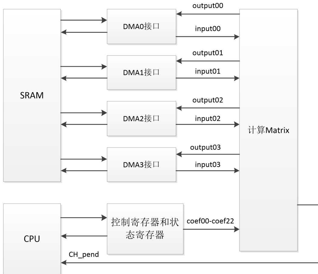
图 4-4 MATRIX Mutiplies 的模块框图
