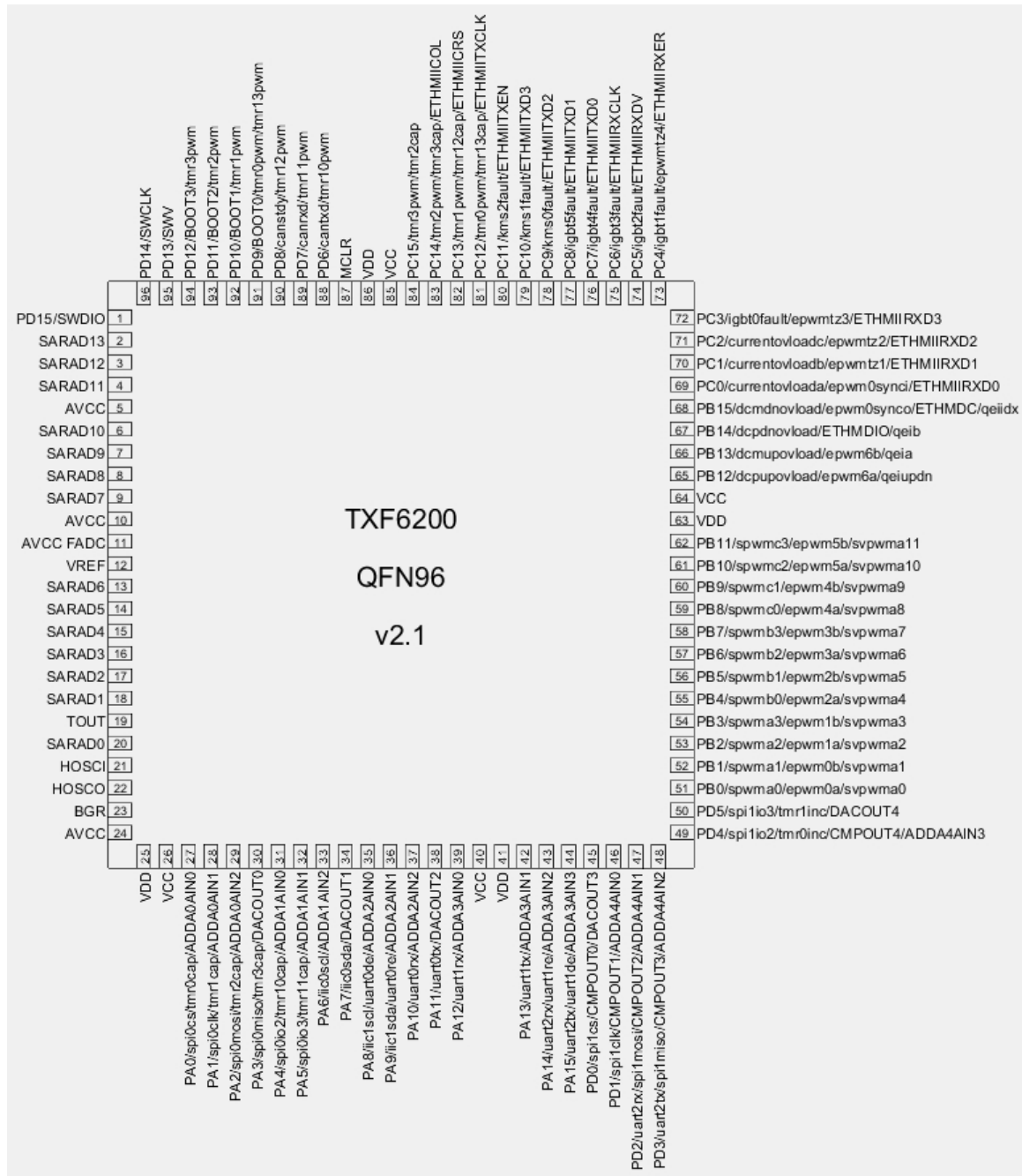
图 3-1 TMF6200 引脚示意图
