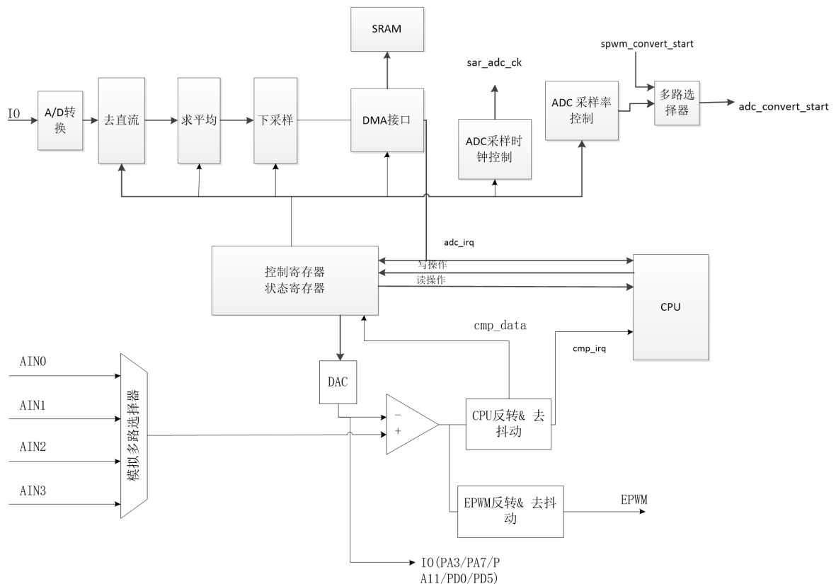
图 8-2 SARADC14~18 框图
