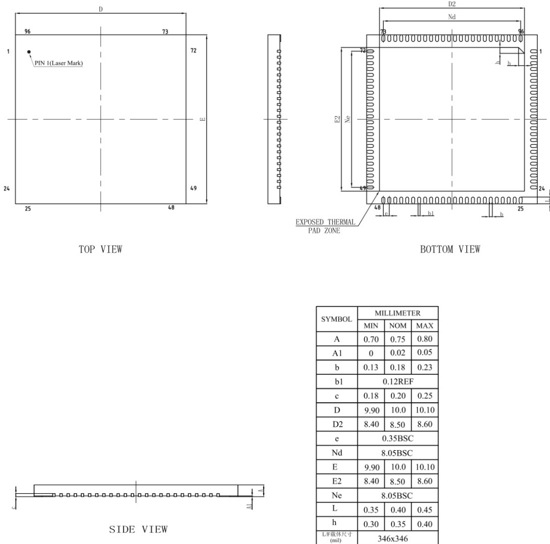
图 3-2 TMF6200 封装图
