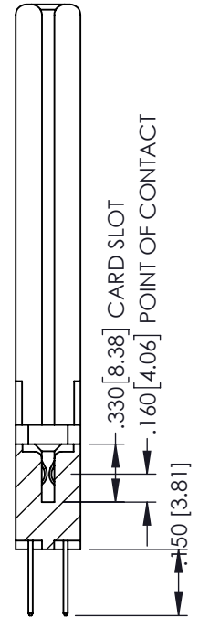
SECTION A-A
