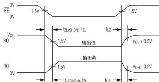
图5：接收器开启与关闭时序
