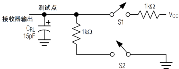
图1：接收器时序测试电路
