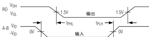
图4：接收器传输延迟
