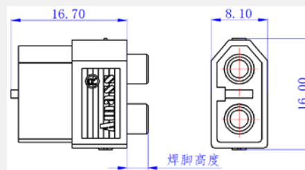
焊脚高度
