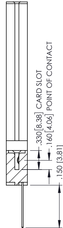
SECTION A-A
