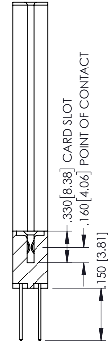
SECTION A-A
