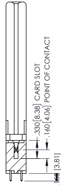
SECTION A-A
