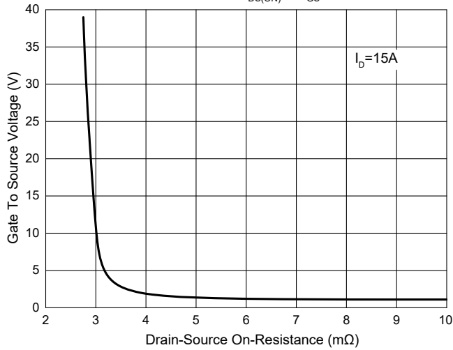
Fig. 3 - R DS(ON) - V GS
