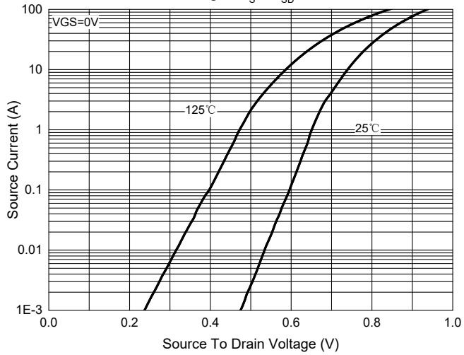
Fig.9 - I_s - V_{SD}
