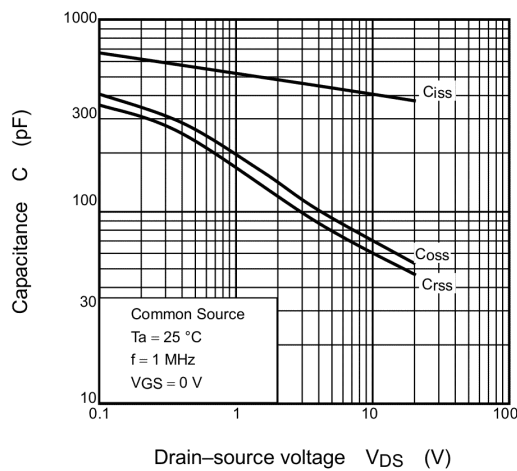
Fig. 7.9 C - V_{DS}
