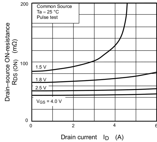
Fig. 7.4 R_{DS(ON)} - I_D
