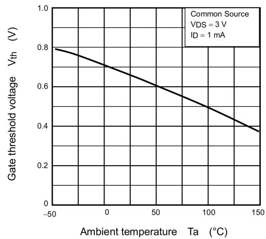
Fig. 7.6 V_{th} - T_a
