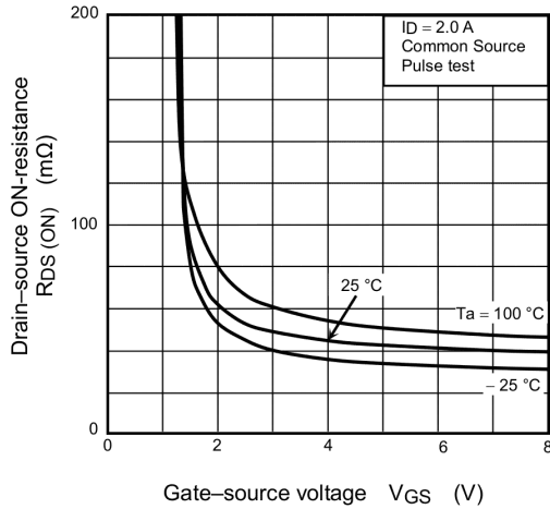
Fig. 7.3 R_{DS(ON)} - V_{GS}
