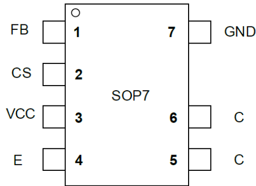
图 2 管脚封装图
