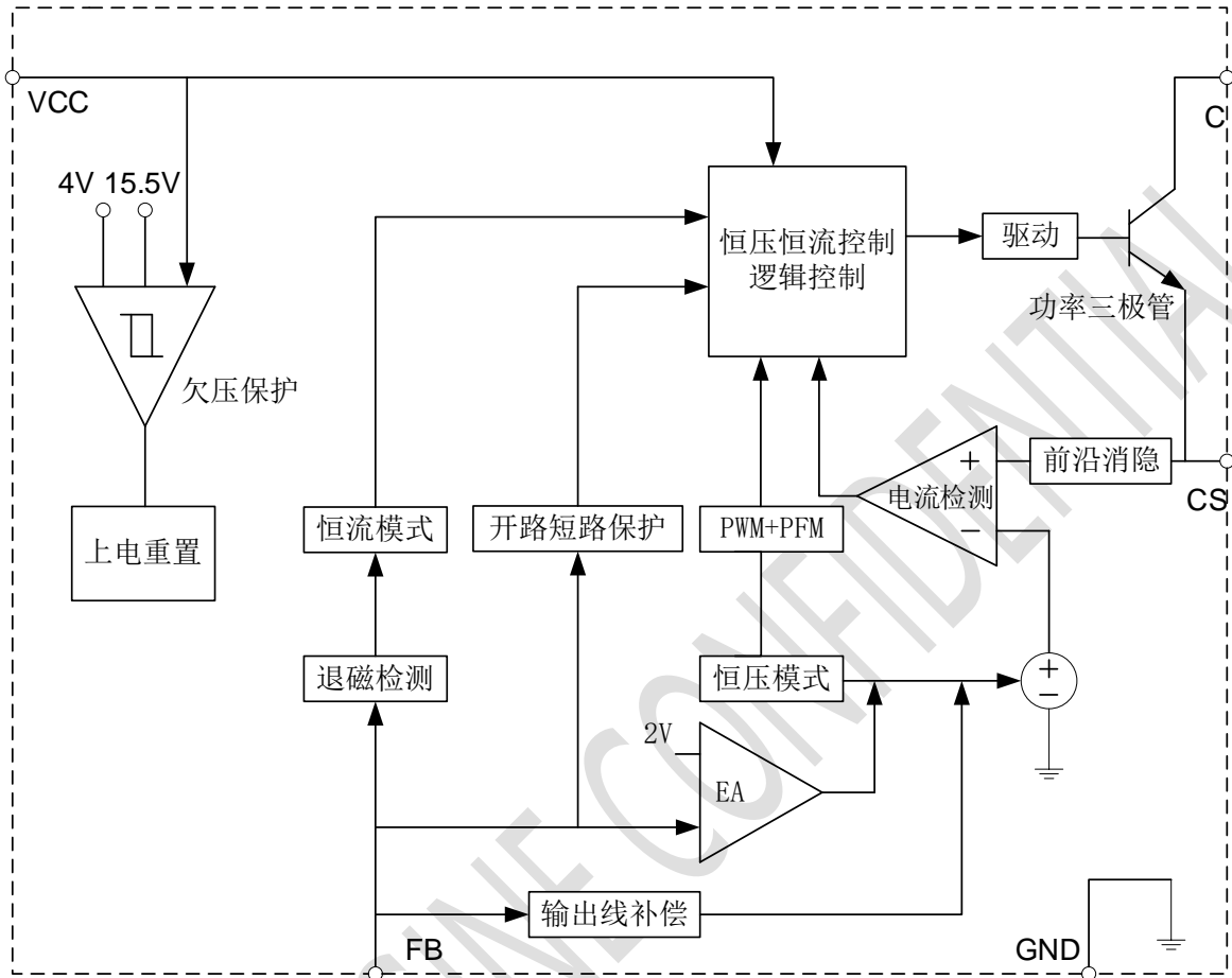
图3 SZ3773C 内部框图
