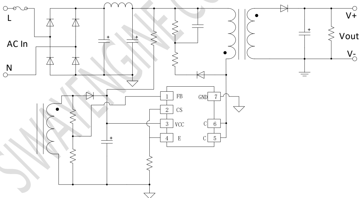
图 1 S3773C 典型应用图
