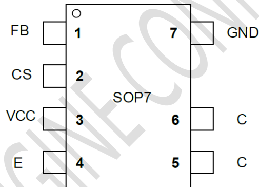
图 2 管脚封装图
