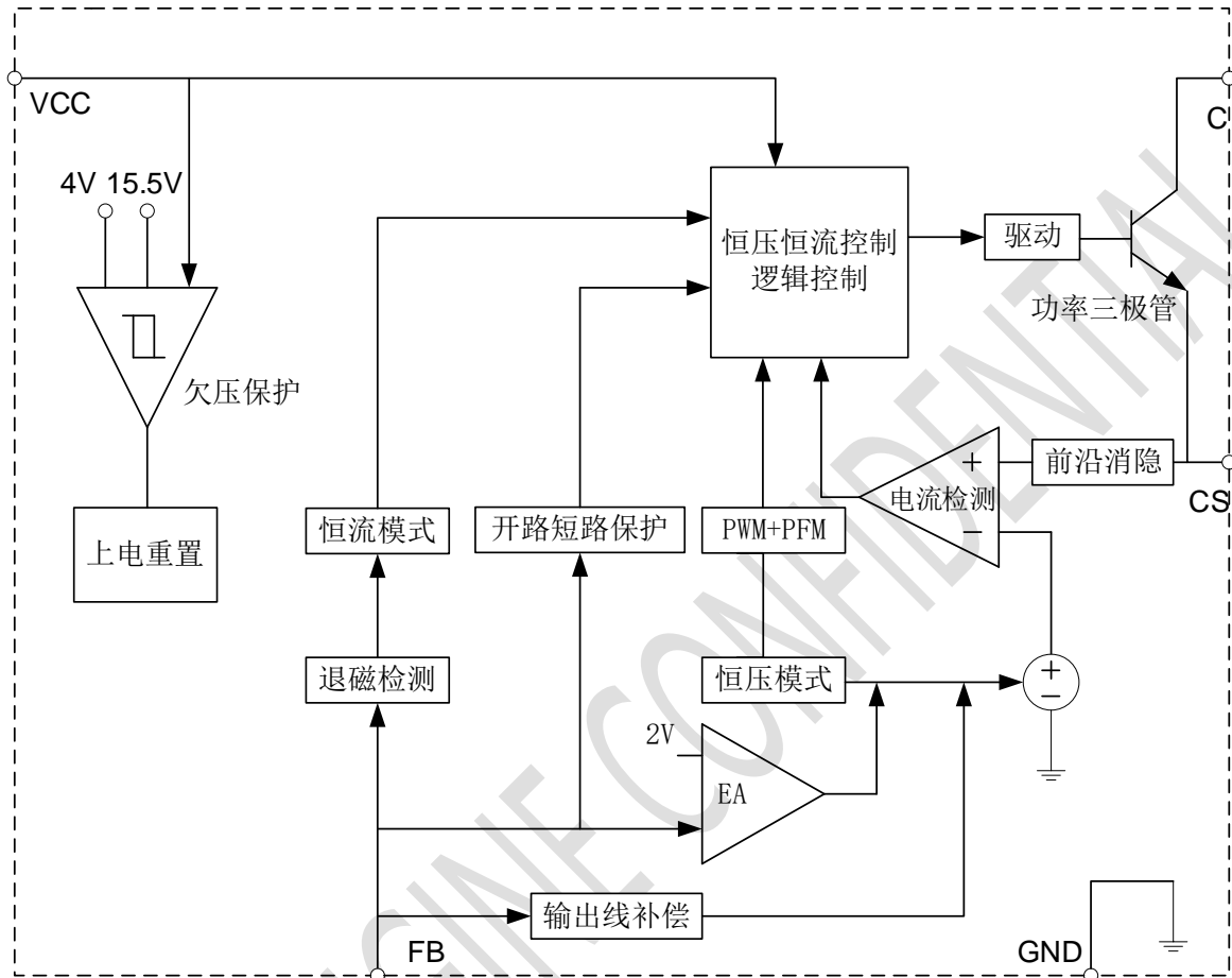
图 3 S3773C 内部框图
