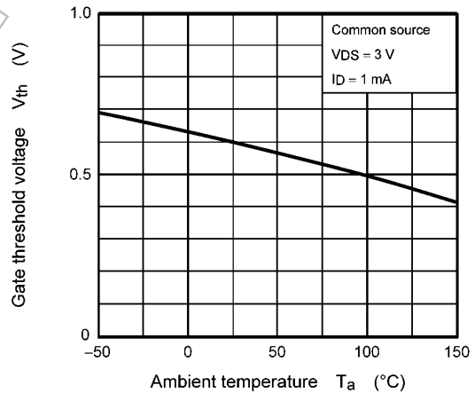
Fig. 8.6 Vth - Ta
