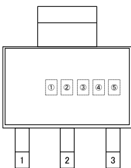
SOT-223
