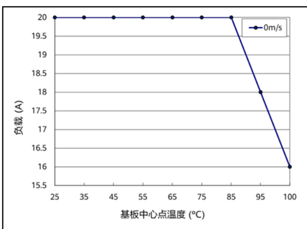
基板热降额曲线 (有散热器)
