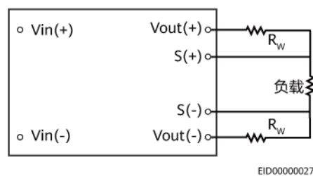
图 5-4 S(+)/S(-)引脚控制原理
