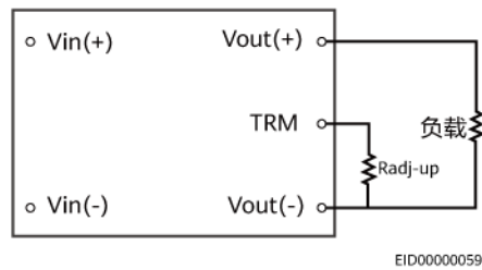
图 5-5 推荐输出电压上调控制原理
