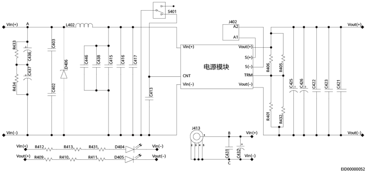
图 4-2 测试电路图
