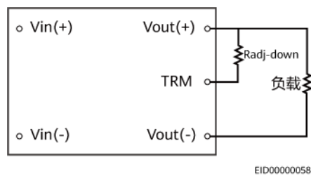
图 5-6 推荐输出电压下调控制原理
