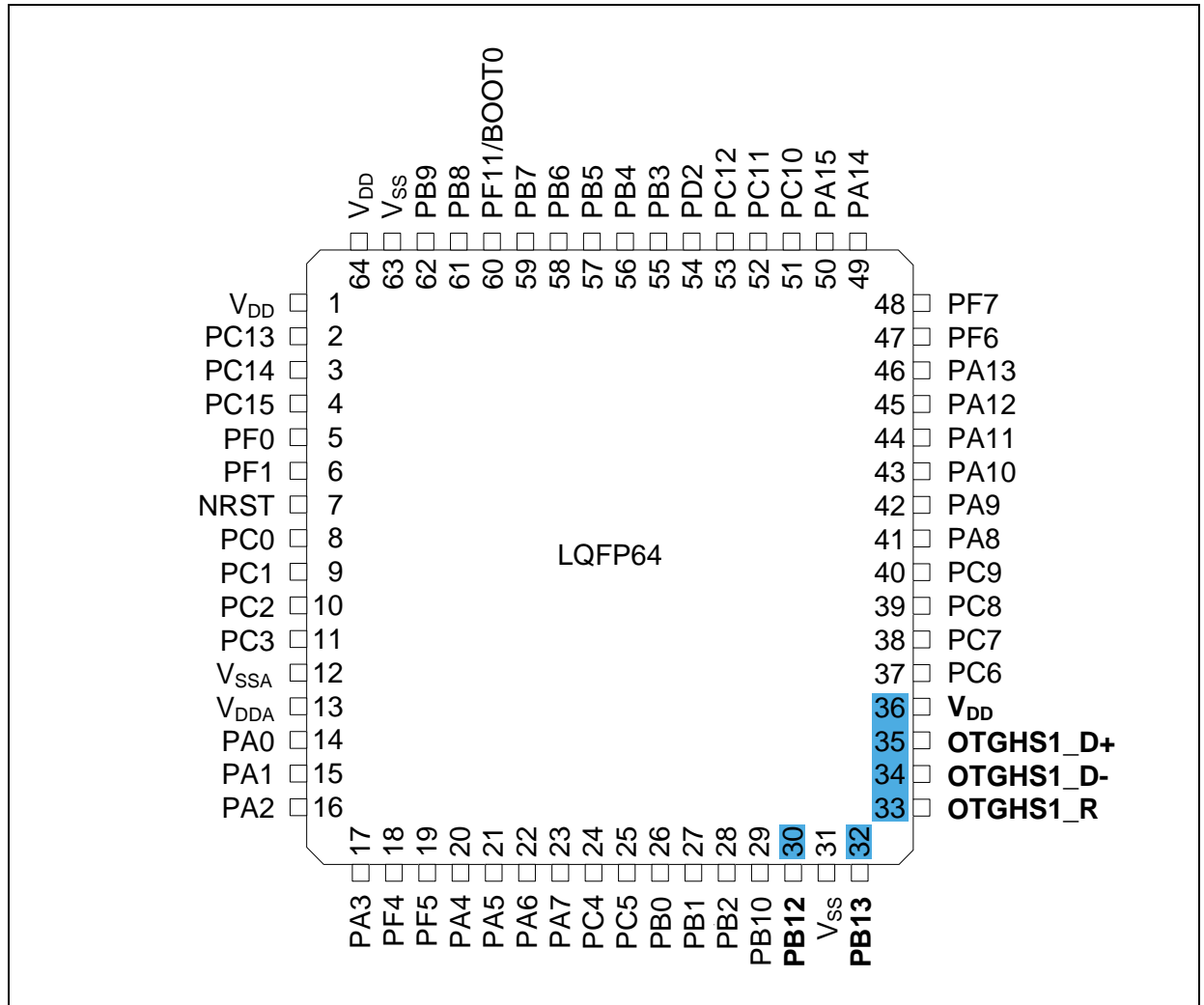
图 1. AT32F405 系列 LQFP64 引脚分布
