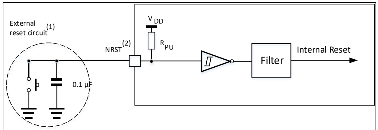
图 19. 建议的 NRST 引脚保护
