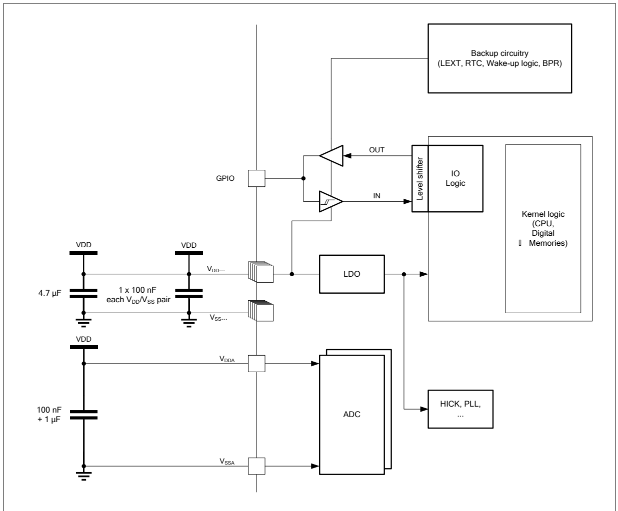
图 9. 供电方案
