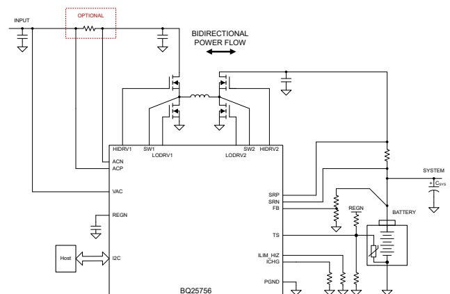
简化原理图
